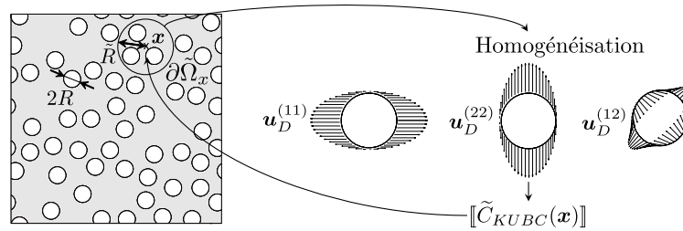
FIGURE 2 – Schéma de la méthode de filtrage (cas KUBC).
