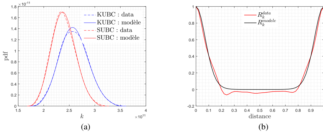
FIGURE 4 – (a) Estimations de la densité du noyau pour de la densité de probabilité du module méso-copique de compressibilité \tilde{k} pour deux conditions aux limites : KUBC (bleu)/SUBC (rouge); (b) Identification de la structure de corrélation R_k avec la fonction cible r (noir, voir Eq. (8)).
