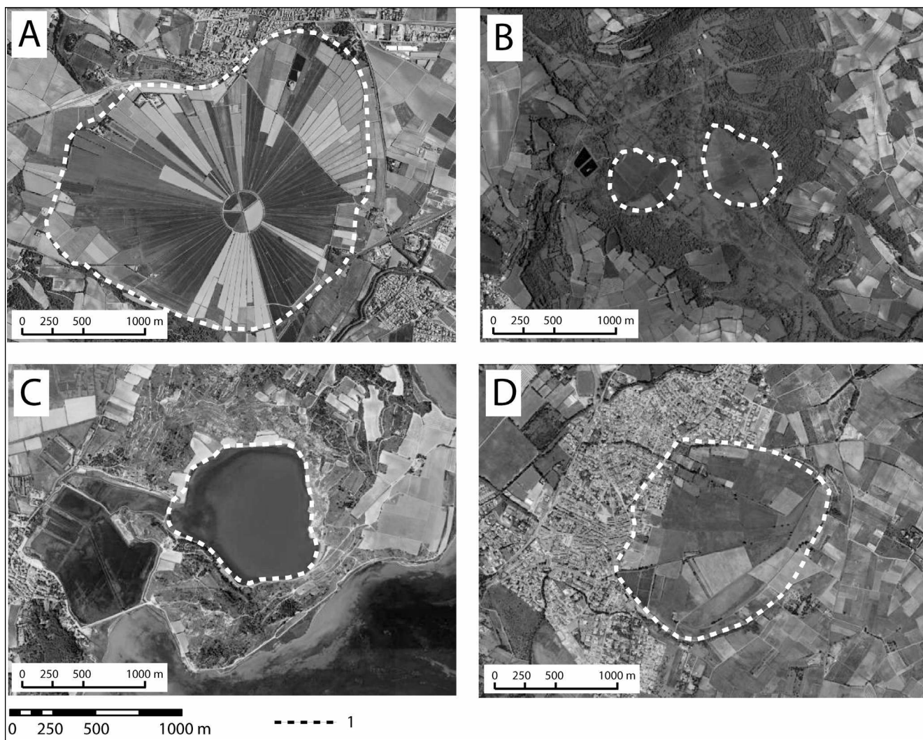
Fig. 10 – Photographies aériennes de quelques dépressions du Languedoc central et du Roussillon (Montady, Caux, Nizas, L'Étang du Dou à Peyriac-de-mer et Canohes, données IGN http://www.geoportail.gouv.fr ). 1 : délimitation de la forme sensu largo. A : Dépression de Montady (g1, réseau parcellaire de drainage radioconcentrique médiéval, Hérault). B : L'Estang à Caux (à gauche : non délimité, Hérault) et Le Clot à Nizas (à droite : g2, Hérault). C : L'Étang du Dou à Peyriac-de-mer (g3, origine diapirique attestée, Aude). D : Dépression de Canohes (g3, Pyrénées-Orientales). Ces formes sont localisées sur la fig. 9.
