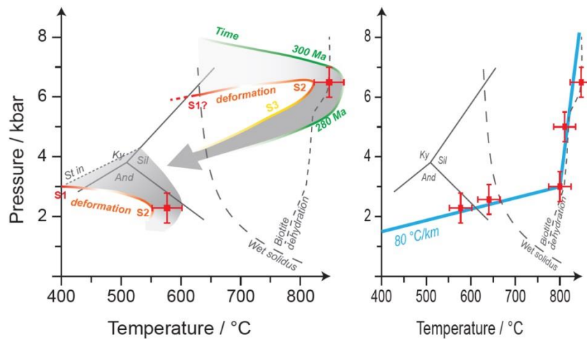
Fig. 2. – À gauche, diagramme pression- température montrant le chemin PTtd des granulites et des micaschistes du massif du St Barthélémy; à droite diagramme pression- température montrant le géotherme à 300 Ma dans ce même massif (Lemirre, 2018).
