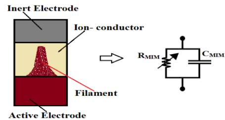
Figure 1. Modélisation d'une cellule MIM
