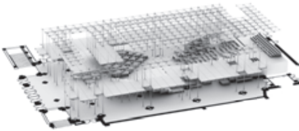
FIG. 6. AXONOMÉTRIE ANALYTIQUE D'UNE HYPOTHÈSE DE RESTITUTION DU PROJET D'AMÉNAGEMENT DU HALL DES BEAUX-ARTS DE LUCIEN-JACQUES BAUCHER. SOURCE : ÉLÉONORE DAVID ET RAPHAËL PADOVANI, FACULTÉ D'ARCHITECTURE LA CAMBRE-HORTA DE L'UNIVERSITÉ LIBRE DE BRUXELLES, 2013.
