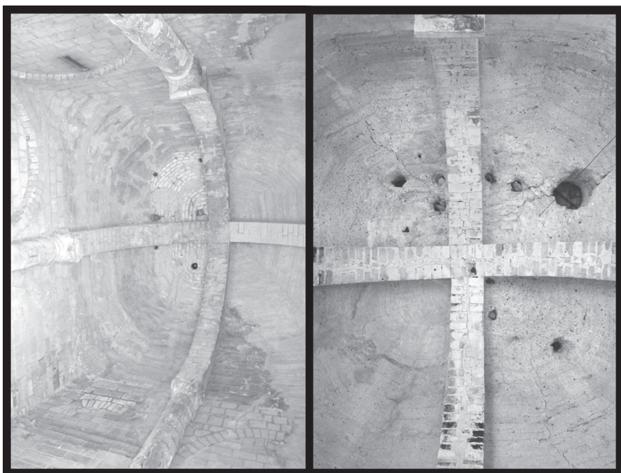
Fig. 6. Coupôles au premier étage de la tour Charlemagne (à gauche) et de la tour Saint-Paul de Cormery (à droite) (© Th. Pouyet).
