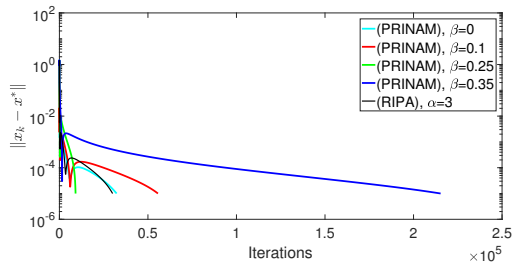
(d) s = 1 , r = 0.5 , q = -0.5
