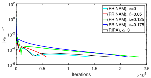
(c) s = 0.5 , r = 0.5 , q = -0.5
