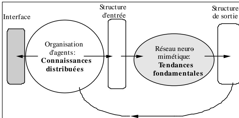
Figure 3. Schéma du couplage organisation d'agents - réseau neuro-mimétique
