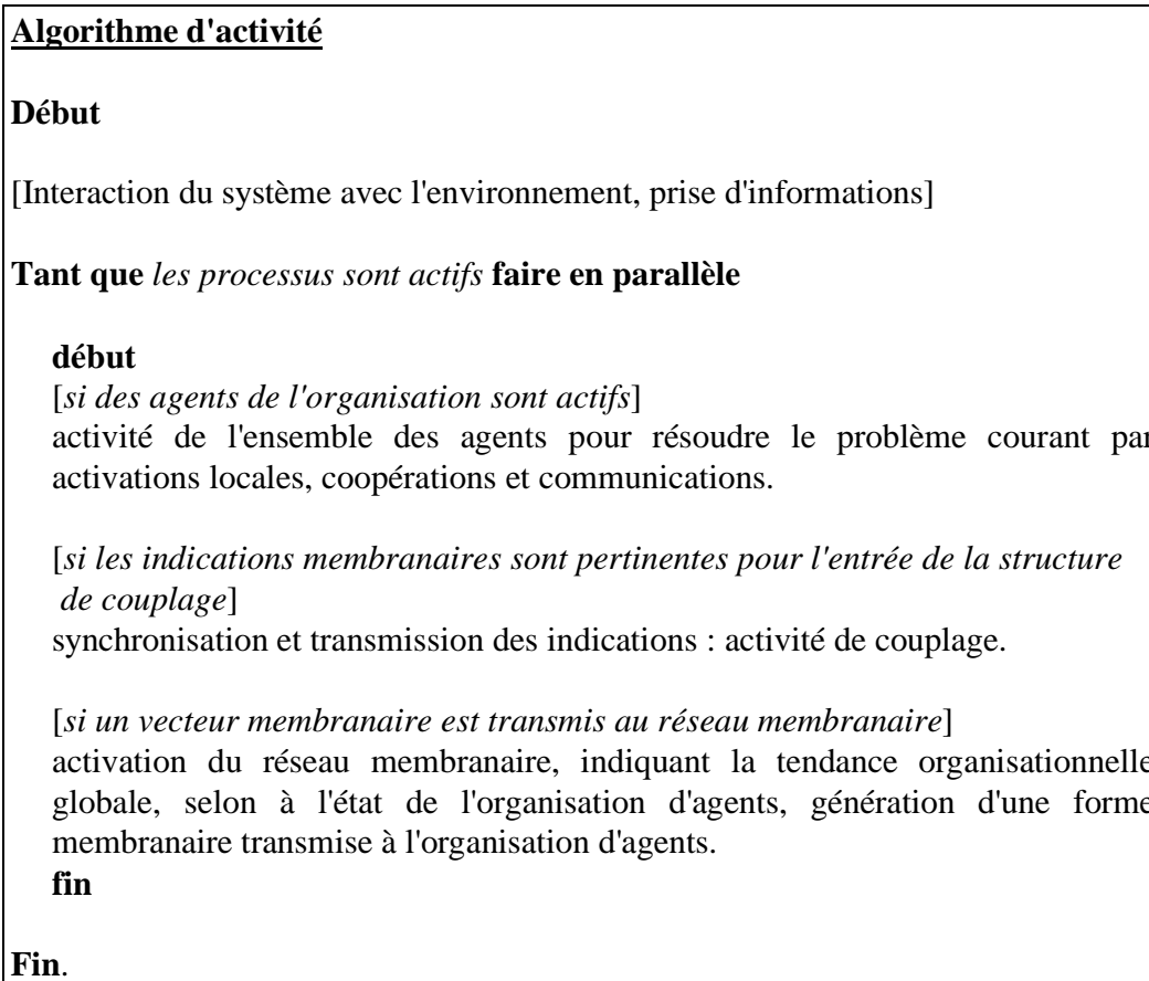
Figure 5. Algorithme d'activité d'un système adaptatif
