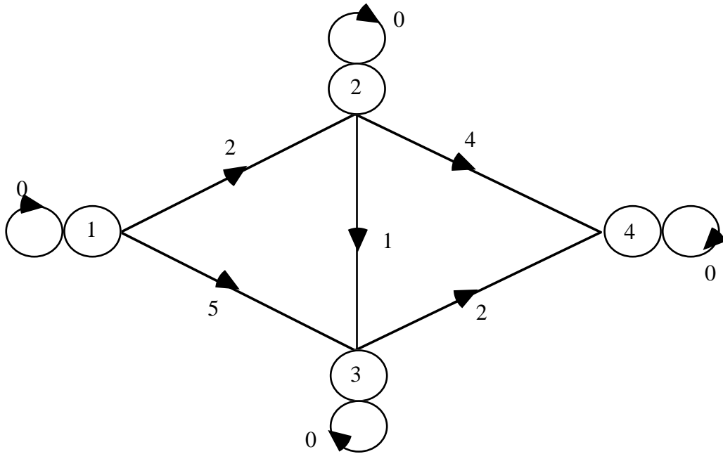
Figure 1 : exemple d'un graphe orienté sur lequel on recherche les longueurs des plus courts chemins d'origine 1. Le vecteur y = (0, 1, 1, 1) est solution du système (1), mais n'est pas solution du problème de plus court chemin d'origine 1 car ce n'est pas la solution minimale de (1).
