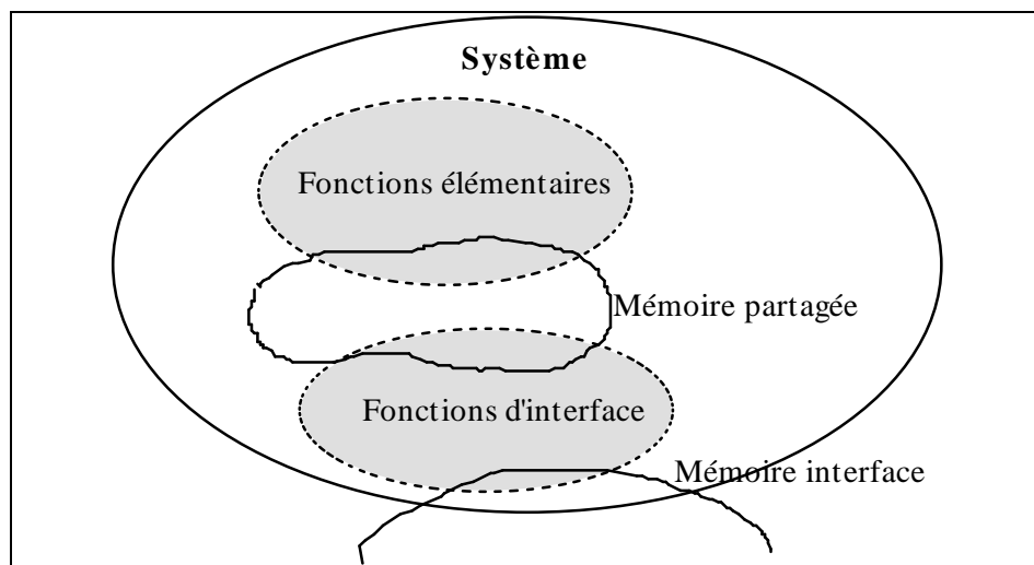
Figure 3. Les fonctions plastiques du niveau fonctionnel.
