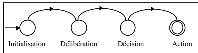
Figure 10. Le macro-automate des agents aspectuels.
