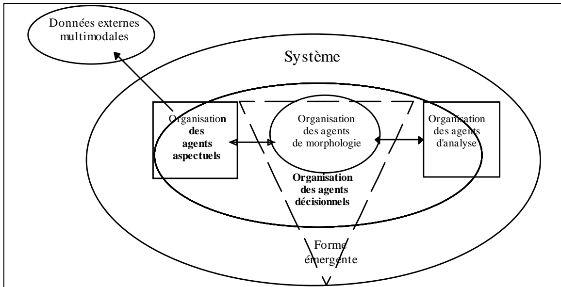
Figure 9. L'architecture du système à quatre organisations d'agents.
