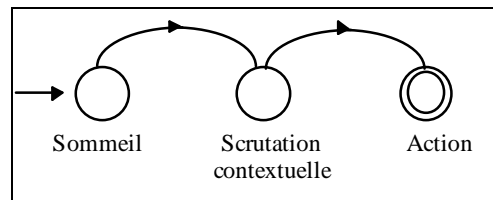
Figure 13. Le macro-graphe d'un agent de morphologie.
