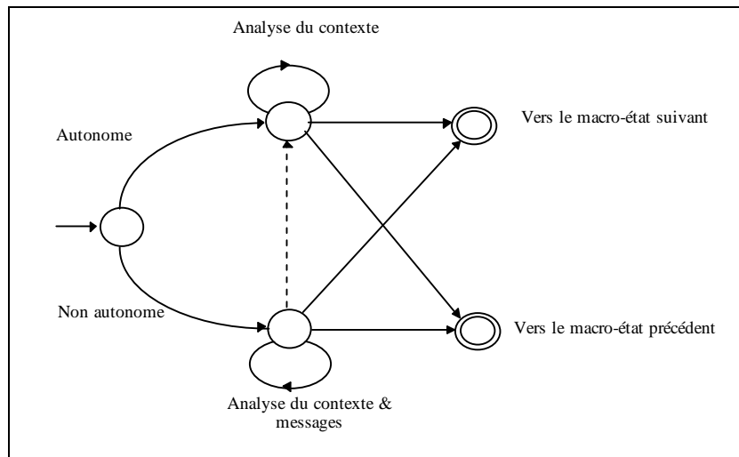
Figure 11. L'ATN de délibération.
