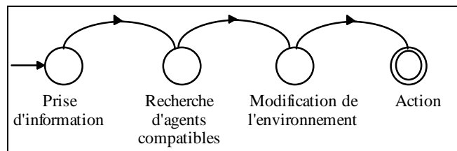
Figure 15. Les quatre macro-états d'un agent d'analyse.
