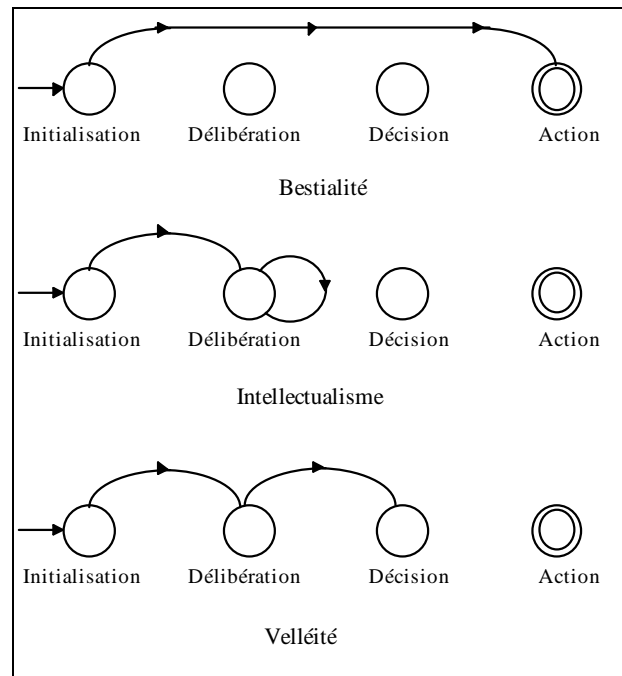
Figure 12. Différentes variations du macro-automate.
