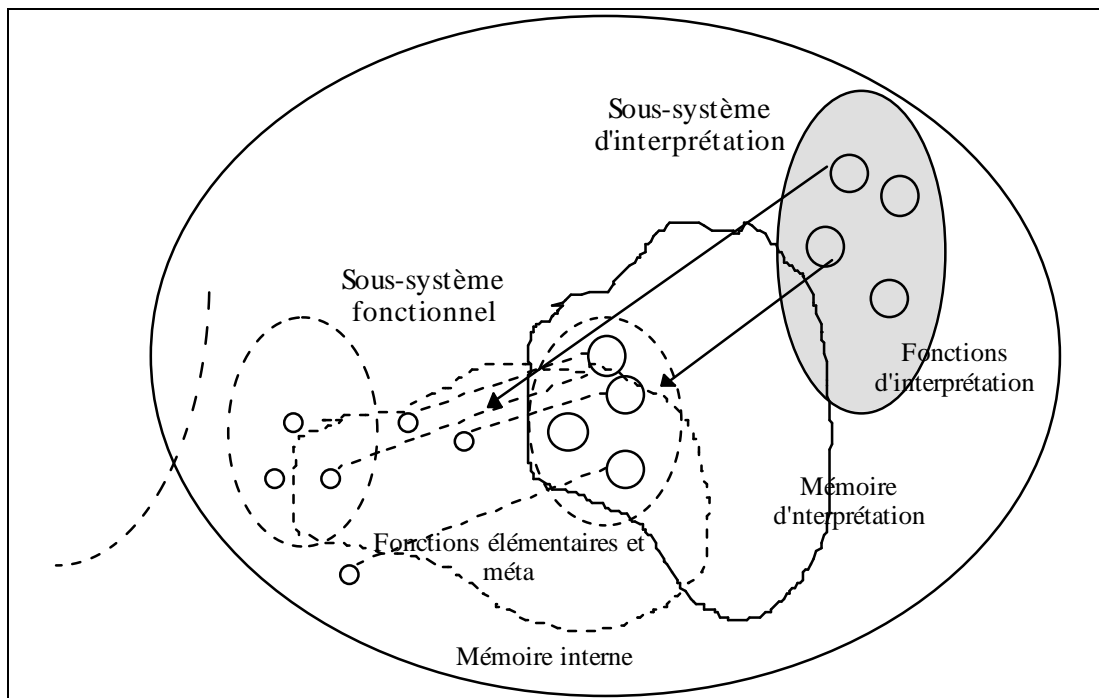
Figure 6. Le système d'interprétation opérant sur les actions du système fonctionnel.
