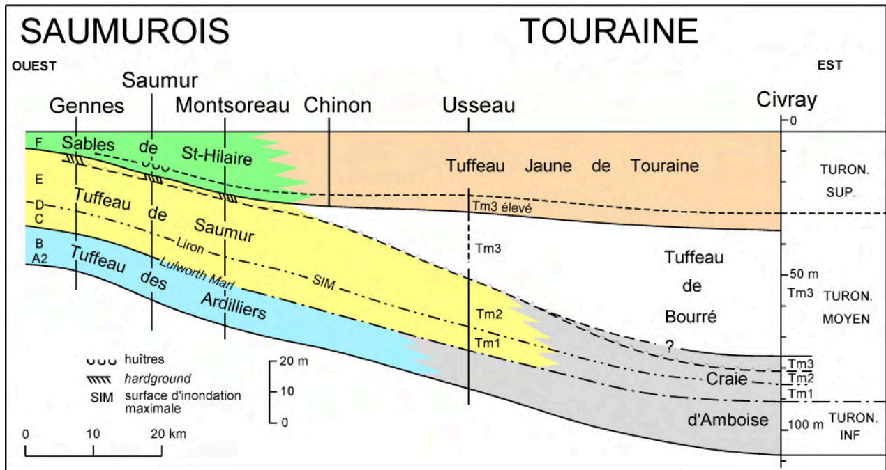
Figure 5 : Relations géométriques entre les formations du Turonien depuis le Saumurois jusqu'à la Touraine (d'après AMÉDRO, MATRION & ROBASYNSKI, coords., 2018, modifié). SIM : Surface d'Inondation Maximale. Geometric relations between Turonian formations from the Saumur area till Touraine area (after AMÉDRO, MATRION & ROBASYNSKI, coords., 2018, modified). SIM: Maximum Flooding Surface (MFS).
