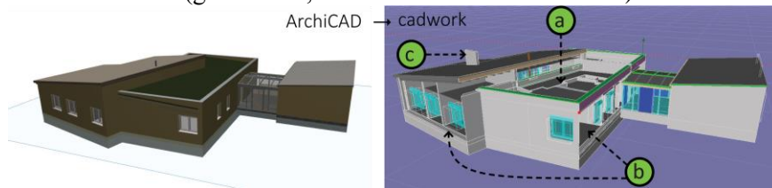
Figure 4: Visualisation du modèle 3D des architectes dans ArchiCAD, et son import dans cadwork. Des toits (a) et murs (b) sont manquants et certains murs (c) ne sont plus coupés par la toiture.
