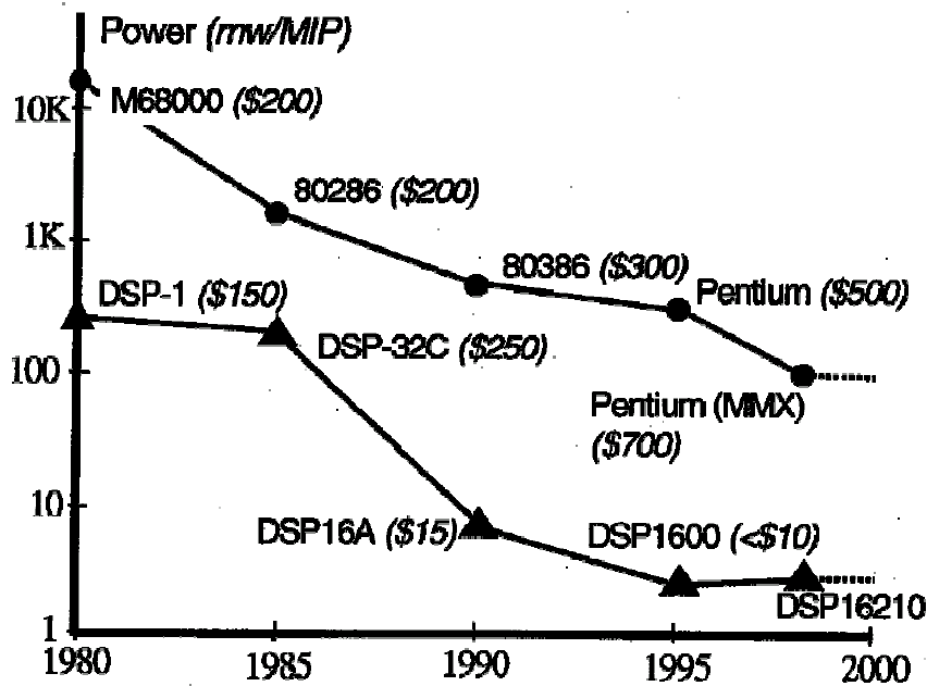
Figure 25 Coût et Consommation des DSPs / Microprocesseurs
