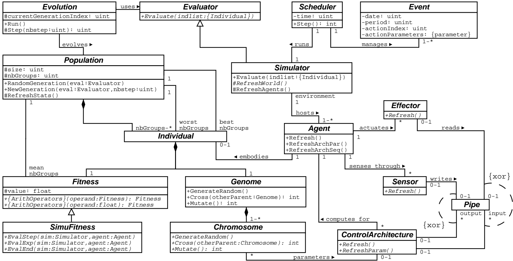
Figure 8. Diagramme des classes de SFERES
