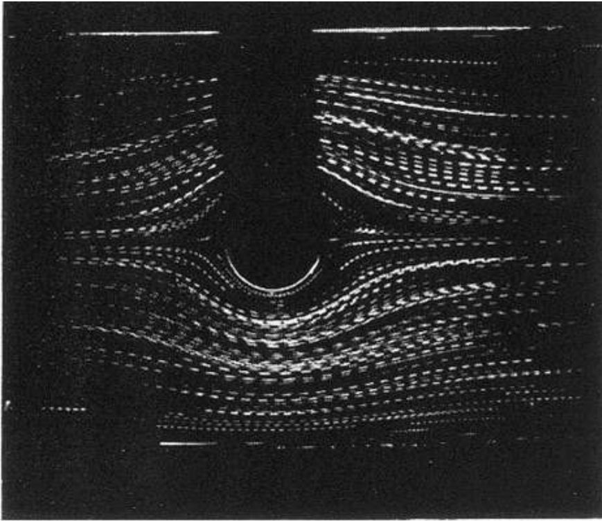
Figure 5 [fichier Crausse1936-45_8PCzoom1.jpg] - Chronophotographie de l'écoulement (de gauche à droite) autour d'un barreau cylindrique (Crausse 1936).
