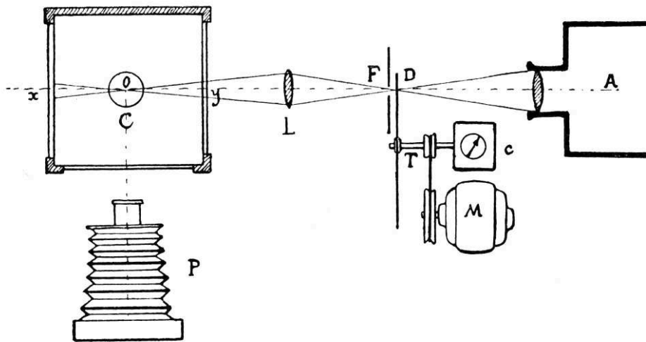
Figures 4 [Fichier CamEsc38_Fig14.jpg] - Montage de chronophotographie : le faisceau lumineux issu de A est intercepté par un disque denté D entraîné en rotation par le moteur M. Le faisceau intermittent sortant de la fente F éclaire un plan diamétral xOy de l'écoulement dans la conduite C, photographié par l'appareil P (Camichel 1920).
