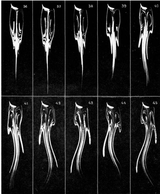
Figure 7 [fichier Dup30_Fig36-45.jpg] - Photographies extraites d'un film montrant le développement d'un sillage ondulant à l'aval d'un barreau cylindrique (Camichel, Dupin et Teissié-Solier 1927).
