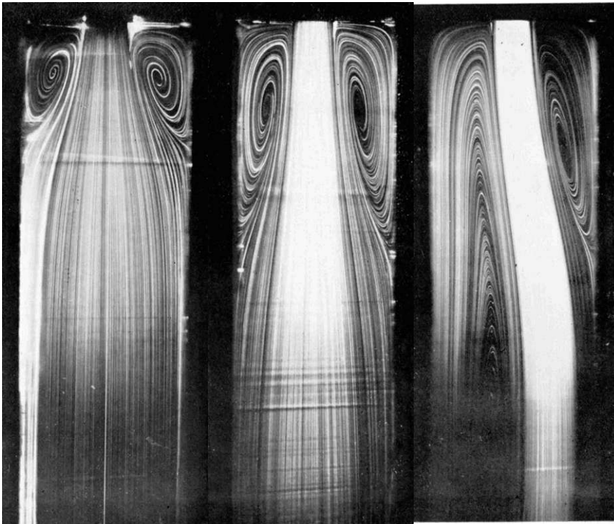
Figure 6 [Fichiers Cam35_Fig9.jpg, Cam35_Fig10.jpg, Cam35_Fig11.jpg] - Écoulement (de haut en bas) à la sortie d'un élargissement brusque. L'écoulement, symétrique à faible vitesse (à gauche), s'oriente vers l'une ou l'autre des parois latérales lorsque la vitesse augmente (à droite) (Camichel 1935).
