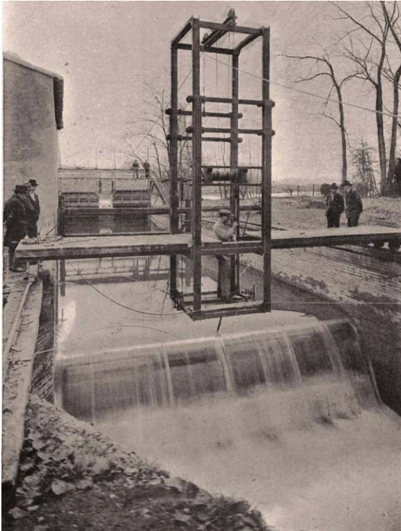
Figure 3 [Fichier ArchIMF_18_13.jpg] - Le canal courbe du Laboratoire de Banlève, et nacelle de mesure du débit à l'aide du déversoir de Bazin.
