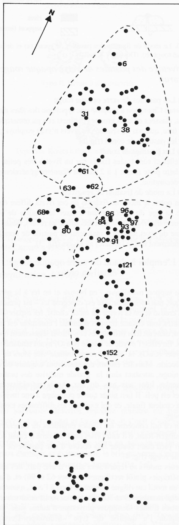
Fig. 5a. Le cimetière de Münsingen-Rain (BE): analyse spatiale du verre opaque rouge et du corail. Le verre opaque rouge.
