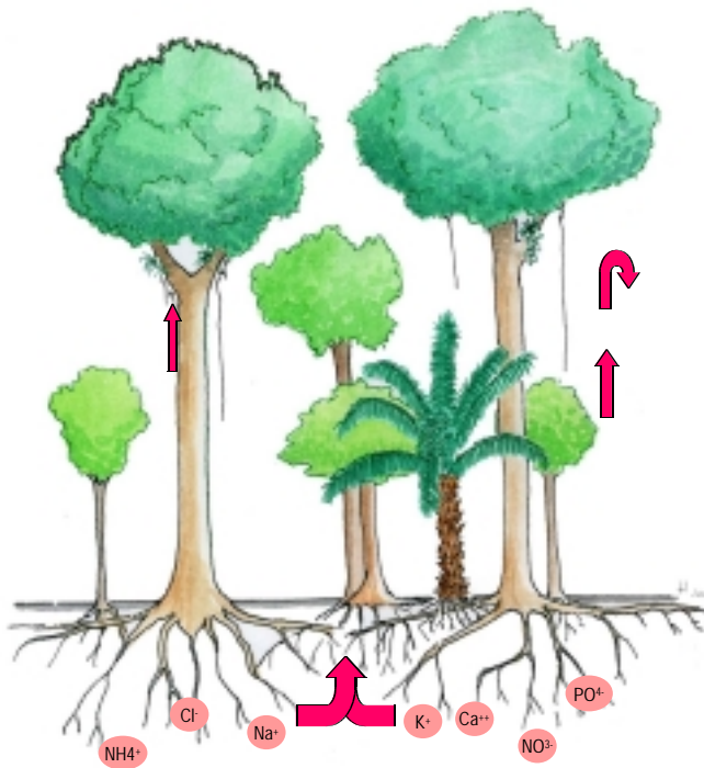
ILLUSTRATION 23 : Régénération de la fertilité d'un sol par une forêt ou une friche arborée
