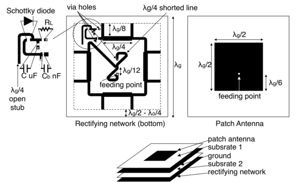
Fig. 1. Rectenna unitcell.
