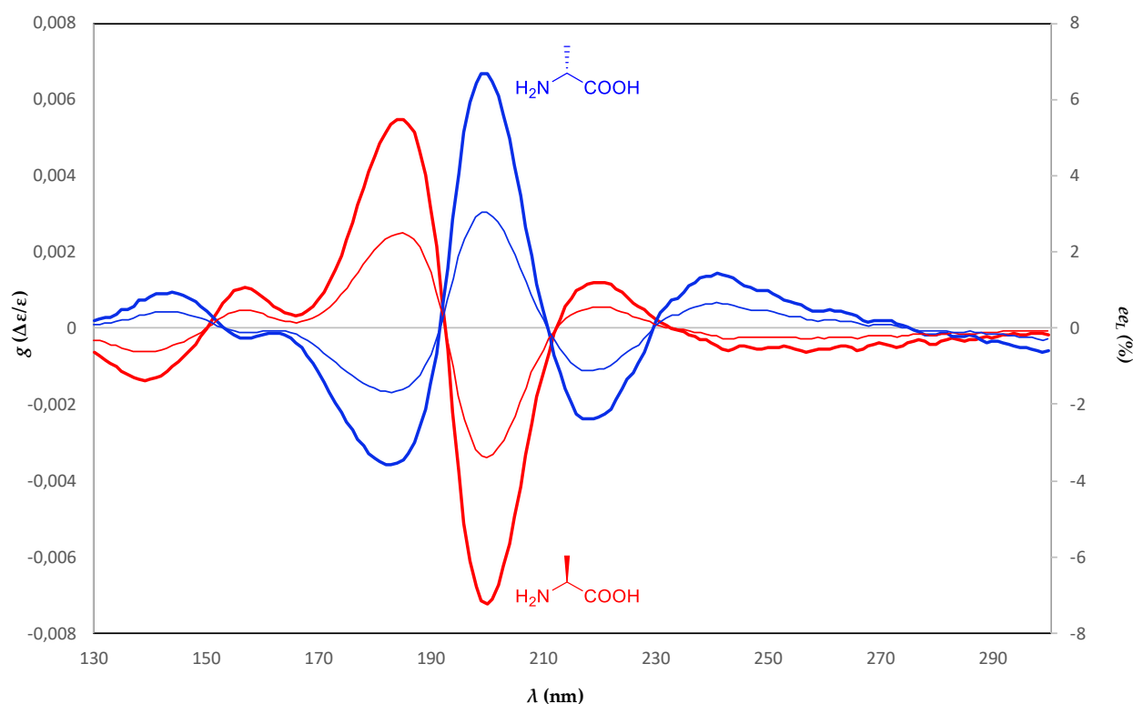
Figure 3 : Spectres d'anisotropie de la L-alanine (ligne rouge épaisse) et de la D-alanine (ligne bleue épaisse) à l'état solide dans l'UV. Les spectres des énantiomères sont opposés et représentatifs de la différence d'absorption de la l- et r-LCP par l'énantiomère. Les lignes bleues
