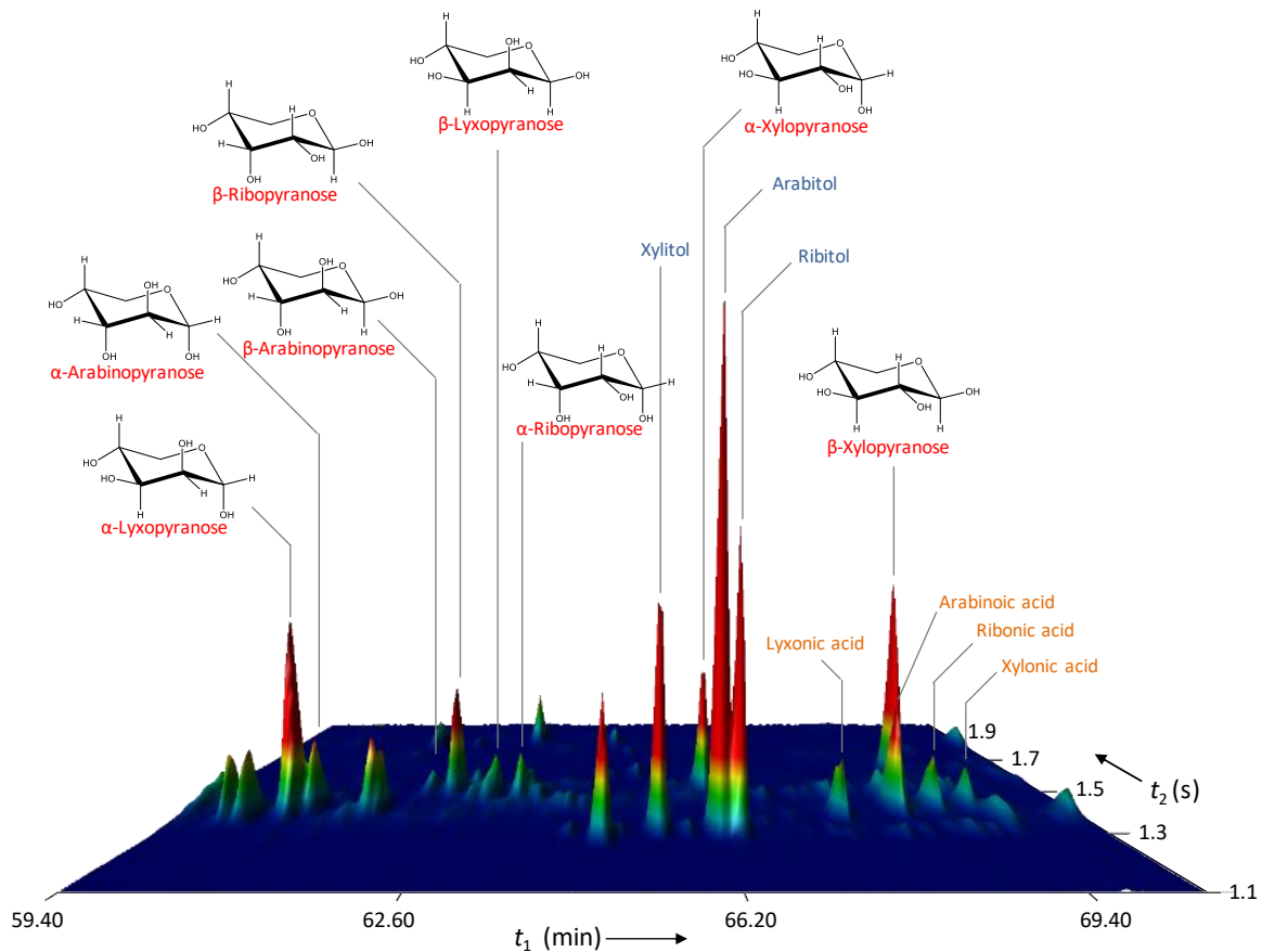
Figure 4 : Chromatogramme bidimensionnel en phase gazeuse du ribose et d'autres sucres simples extraits du résidu organique d'un analogue de glaces interstellaires.
