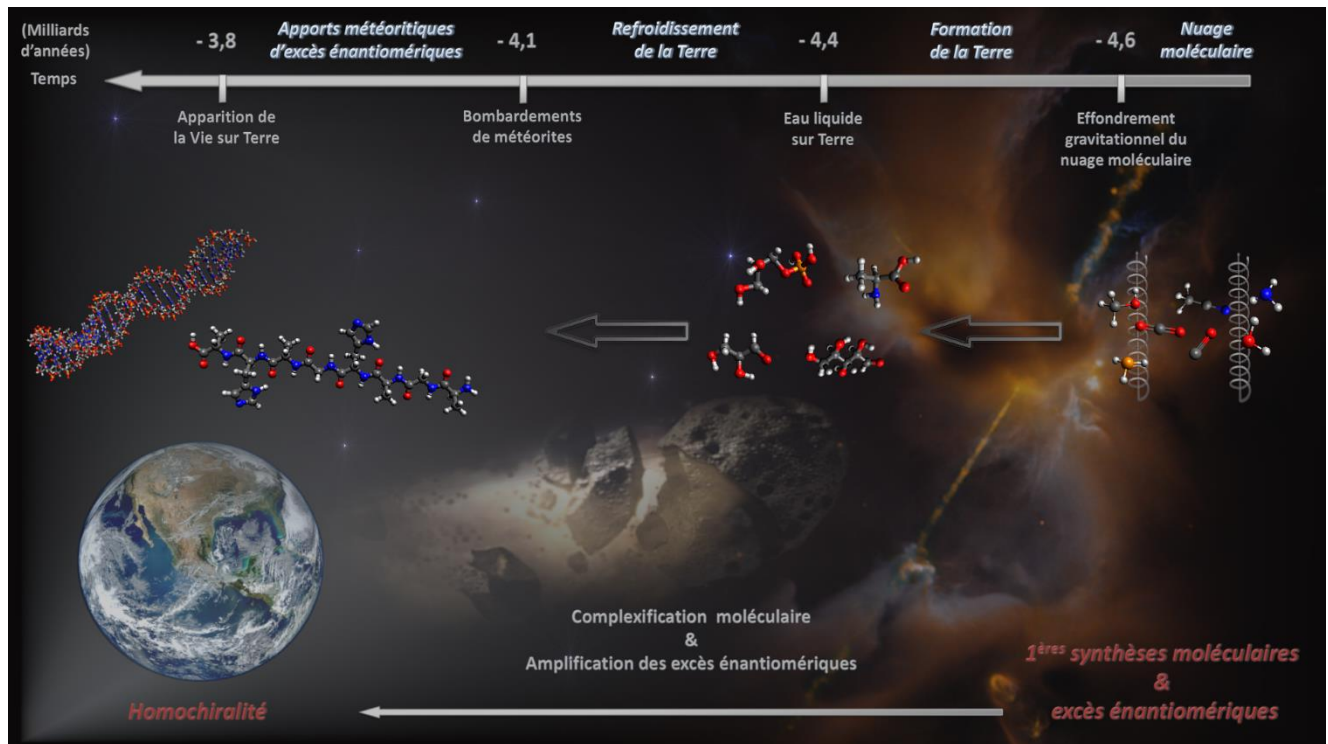
Figure 2 : Synthèse et évolution des premières molécules chirale, par interaction de la LCP dans les nuages moléculaires, menant aux biopolymères.
