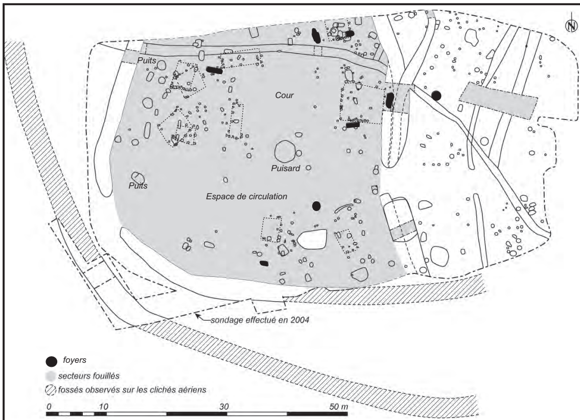
Enclos de métallurgie du fer de Kergroas à Paule (Côtes d'Armor)
