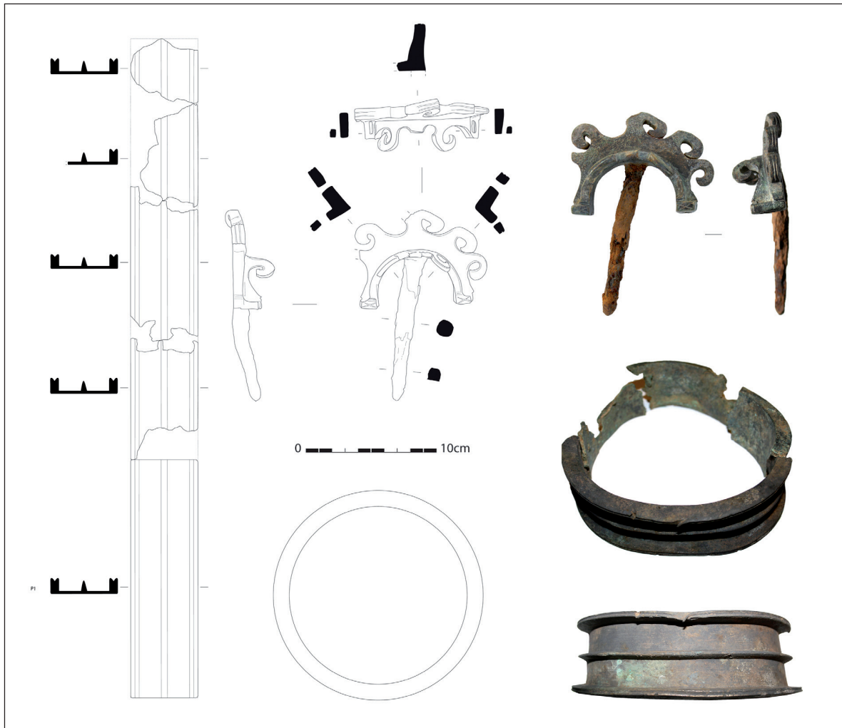
Fig. 2 : Clavette et frette de moyeu de char découvertes en 2012 sur le site du Peillard (Isère). Dessins B. Bourguignon, université Lumière Lyon 2.
