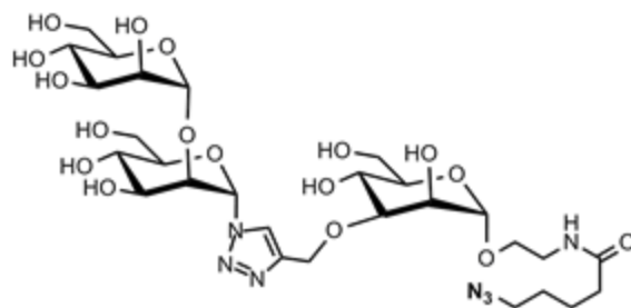
PMan4-azide 6a
