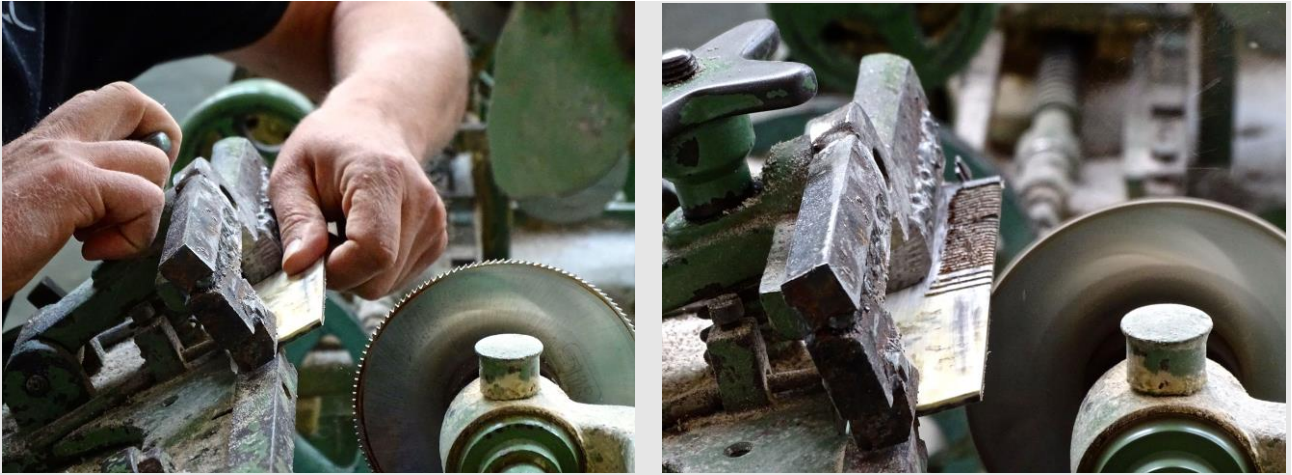
Ill. 3a-b. Mise en place du peigne dans une stadeuse (entreprise Azéma-Bigou). © Mathilde Lamothe, 16 mai 2019.
