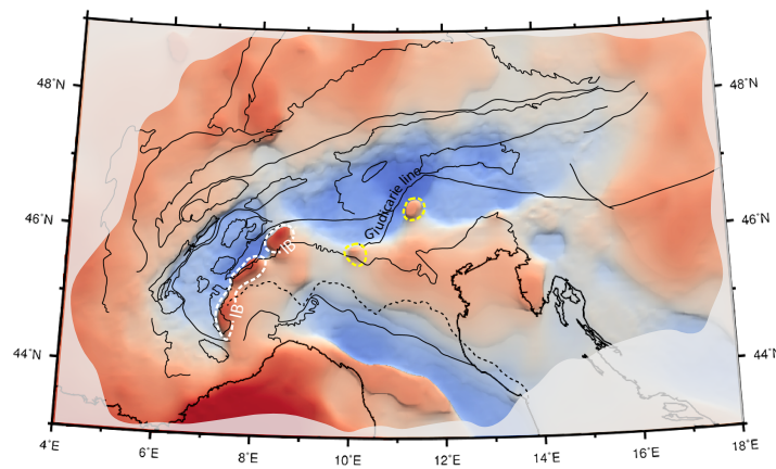
(b) Iso- V_s depth map (4.0 km/s)
