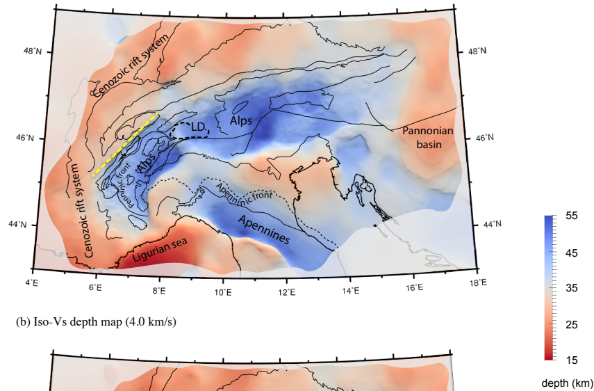
(a) Iso- V_s depth map (4.2 km/s)
