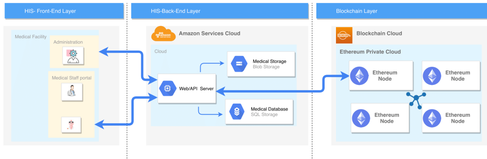
FIG. 1 – Architecture de la solution proposée (SIS et BiiMED).
