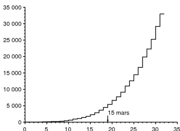
Рисунок 1. а) Совокупное количество случаев, выявленных во Франции в период с 25 февраля по 27 марта 2020 года, согласно данным Santé publique France. б) натуральный логарифм совокупного числа случаев и линий линейной регрессии.
