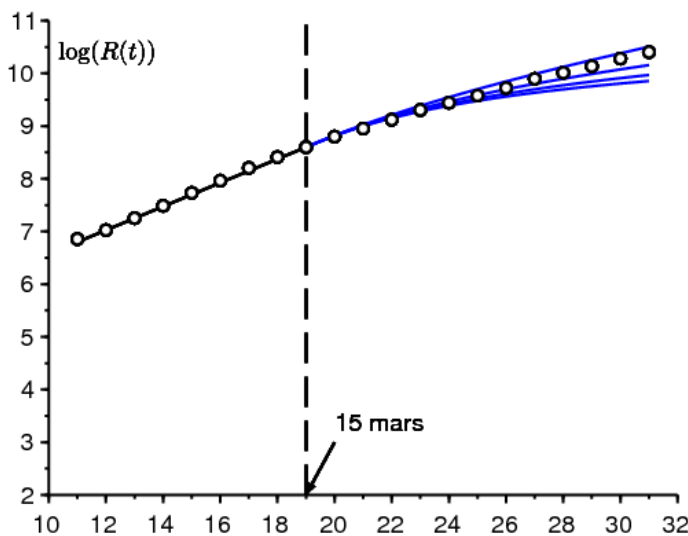
Рисунок 4. Натуральный логарифм числа случаев между 7 и 27 марта (маленькие кружки) и \log(R(t)) как функция времени t в 4 симуляциях сверху вниз q \in \{1,5; 2; 2,5; 3\} ,
