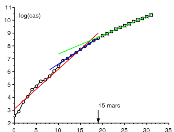
Рисунок 1. а) Совокупное количество случаев, выявленных во Франции в период с 25 февраля по 27 марта 2020 года, согласно данным Santé publique France. б) натуральный логарифм совокупного числа случаев и линий линейной регрессии.
