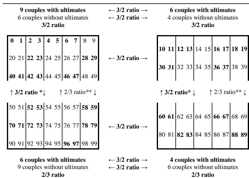
Fig.18 Strong entanglement of the distribution of 25 couples with ultimates and of 25 couples without ultimate in the matrix of the first hundred numbers. Ratios between couples respectively with ultimates* and without ultimate**. Forte intrication de la distribution des 25 couples avec ultimes et des 25 couples sans ultime dans la matrice des cent premiers nombres. Ratios entre couples respectivement avec ultimes* et sans ultimes**.
