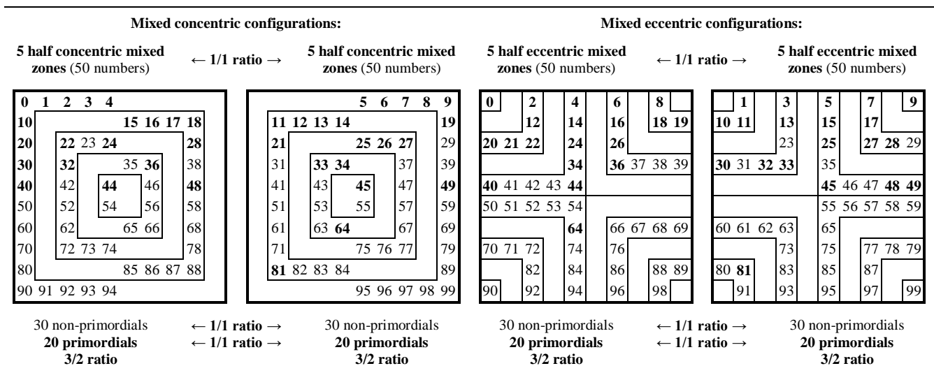
Fig. 46 From the matrix of the first hundred numbers, concentric and eccentric mixed configurations of sub-matrices to 50 entities each opposing their non-primordials and their primordials in 1/1 ratios. Depuis la matrice des cent premiers nombres, configurations concentriques et excentriques mixtes de sous matrices de chacune 50 entités opposant leurs non primordiaux et leurs primordiaux en ratios 1/1.
