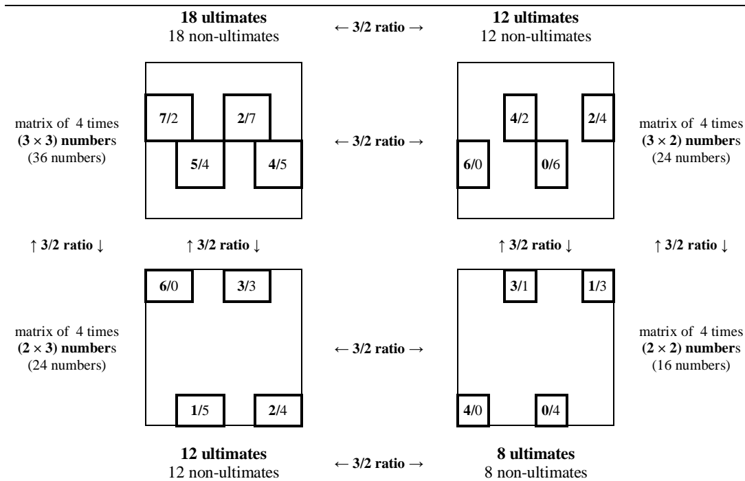
Fig. 30 Four sub-matrices of ten Fibonacci sequences with equal distribution of the ultimate and non-ultimate numbers and 3/2 transcendent ratios. See Fig. 24 and 29. Quatre sous matrices des dix suites de Fibonacci avec égale distribution des nombres ultimes et non ultimes et ratios 3/2 transcendants. Voir fig. 24 et 29.
