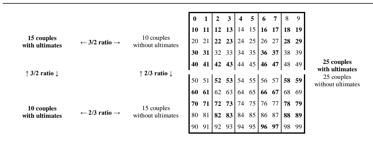
Fig.17 Distribution of the 25 couples with ultimates and the 25 couples without ultimates in the matrix of the first hundred numbers. Distribution des 25 couples avec ultimes et des 25 couples sans ultime dans la matrice des cent premiers nombres.
