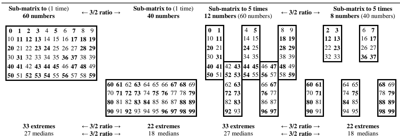
Fig. 53 Distribution of the numbers to extreme and median classes in two little diluted and more diluted double sub-matrices of the first 100 numbers. Distribution des nombres de classes extrêmes et médianes dans deux doubles sous matrices peu diluées et plus diluées des 100 premiers nombres.
