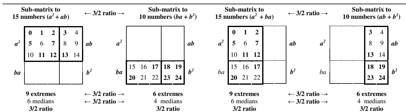
Fig. 56 Distribution of the numbers to extreme and median classes in two double sub-matrices of the first 25 numbers. Configurations inferred from the identity (a + b)^2 = a^2 + 2ab + b^2 where a and b have the values 3 and 2.. Distribution des nombres de classes extrêmes et médianes dans deux doubles sous matrices des 25 premiers nombres. Configurations déduites de l'identité (a + b)^2 = a^2 + 2ab + b^2 où a et b ont les valeurs 3 et 2.
