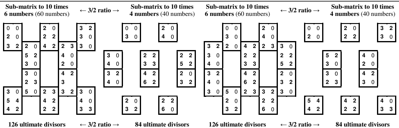
Fig. 50 Respective quantities of the ultimate divisors constituting the first hundred numbers. See matrix in figure 47. Quantités respectives des diviseurs ultimes constituant les cent premiers nombres. Voir matrice figure 47.
