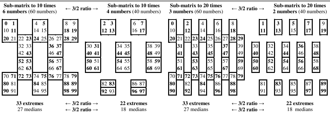
Fig. 54 Distribution of the numbers to extreme and median classes in two diluted and very diluted double sub-matrices of the first 100 numbers. Distribution des nombres de classes extrêmes et médianes dans deux doubles sous matrices diluées et très diluées des 100 premiers nombres.
