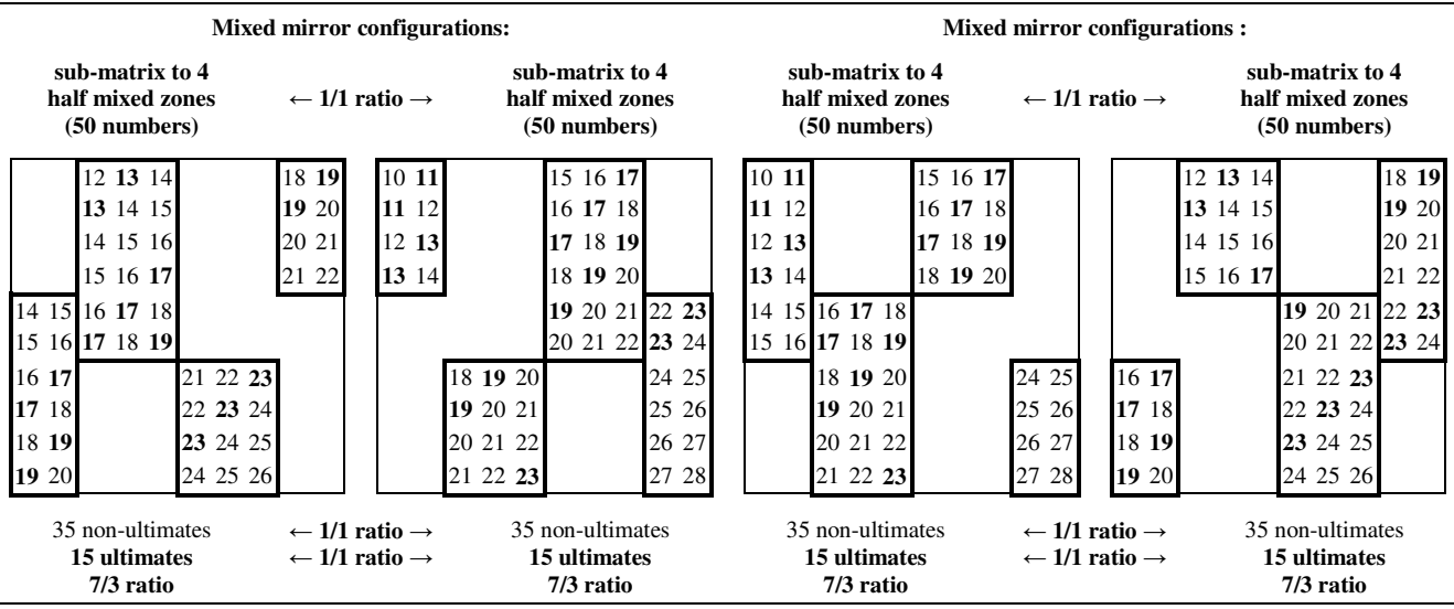
Fig.12 Mixed sub-matrices mirror of addition of the twenty fundamental numbers to 50 versus 50 numbers. Sous matrices mixtes miroir d'additions des vingt nombres fondamentaux de 50 contre 50 nombres.
