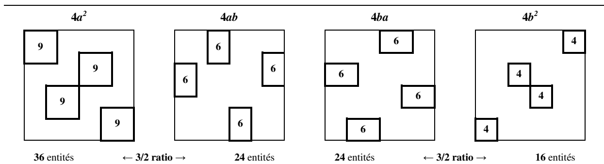
Fig. 26 Recombination of four sub-matrices of 36 → 24 → 24 → 16 entities deduced from the remarkable identity (a + b)^2 = a^2 + 2ab + b^2 . Recombinaison de quatre sous matrices de 36 → 24 → 24 → 16 entités déduite de l'identité remarquable (a + b)^2 = a^2 + 2ab + b^2 .
