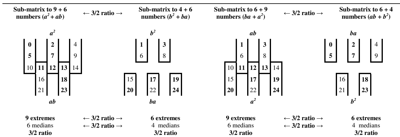
Fig. 58 Distribution of the numbers to extreme and median classes in two double sub-matrices of the first 25 numbers. Configurations inferred from the identity (a + b) \dots . Distribution des nombres de classes extrêmes et médianes dans deux doubles sous matrices des 25 premiers nombres. Configurations déduites de l'identité (a + b) \dots .
