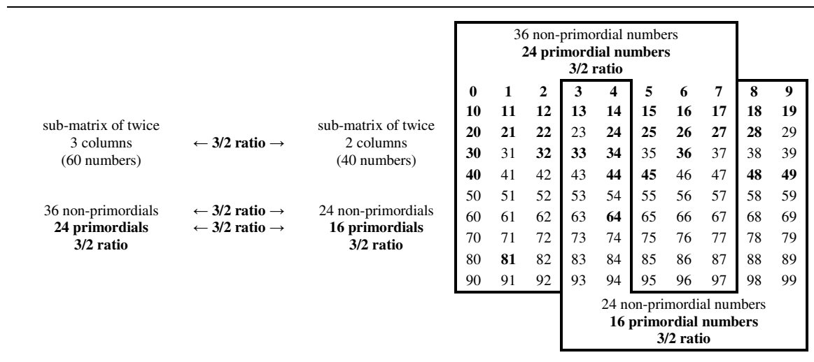
Fig. 41 Distinction and distribution of the 40 primordial and 60 non-primordial numbers in the matrix of the first hundred numbers. Distinction et répartition des 40 nombres primordiaux et 60 non primordiaux dans la matrice des cent premiers nombres.
