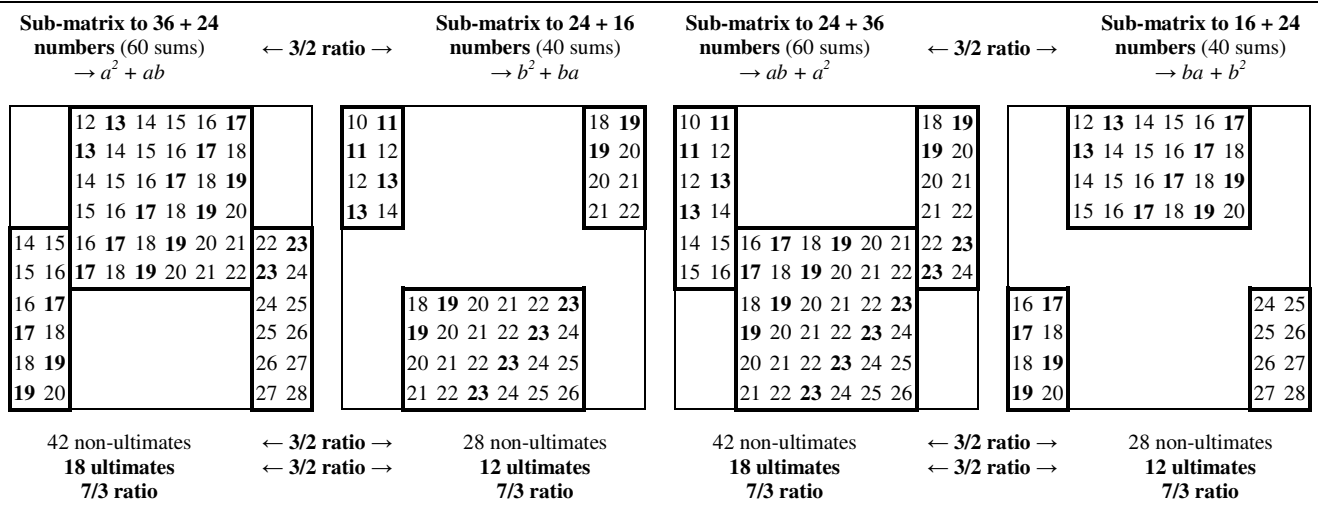
Fig.11 Addition sub-matrices of the twenty fundamental numbers on 60 versus 40 numbers. Geometric variant of the remarkable identity (a + b)^2 = a^2 + 2ab + b^2 . Sous matrices d'addition des vingt nombres fondamentaux de 60 contre 40 nombres. Variante géométrique de l'identité remarquable (a + b)^2 = a^2 + 2ab + b^2
