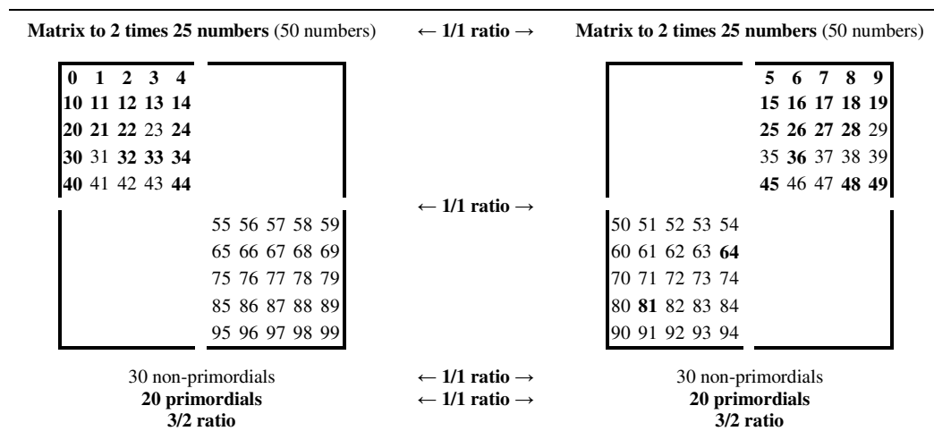
Fig. 42 Equal distribution of the 60 non-primordials and 40 primordials in two sub-matrices of the first hundred numbers. Egale répartition des 60 non primordiaux et 40 primordiaux dans deux sous matrices des cent premiers nombres.
