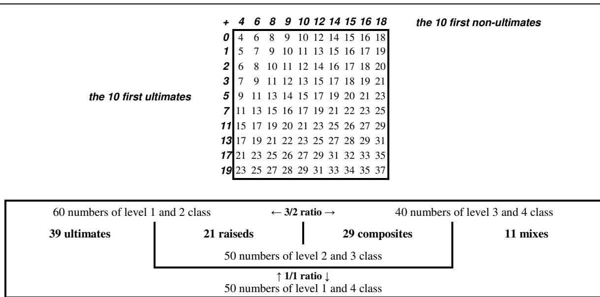
Fig. 67 Distribution of the 4 classes of numbers generated from the additions matrix of the 20 fundamentals segregated into 10 ultimates versus 10 non-ultimates. (See also fig. 37 and 47). Distribution des 4 classes de nombres générés depuis la matrice des additions des 20 fondamentaux ségrégés en 10 ultimes contre 10 non ultimes. (Voir aussi fig. 37 et 47).
