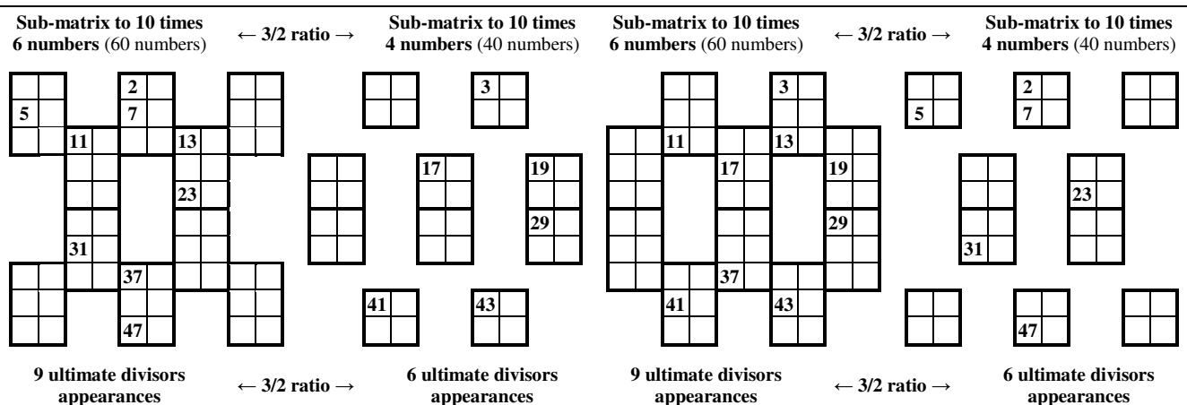
Fig. 51 Distribution of the first appearance of the 15 ultimate divisors in the matrix of the first 100 numbers. Distribution de la première apparition des 15 diviseurs ultimes dans la matrice des 100 premiers nombres.
