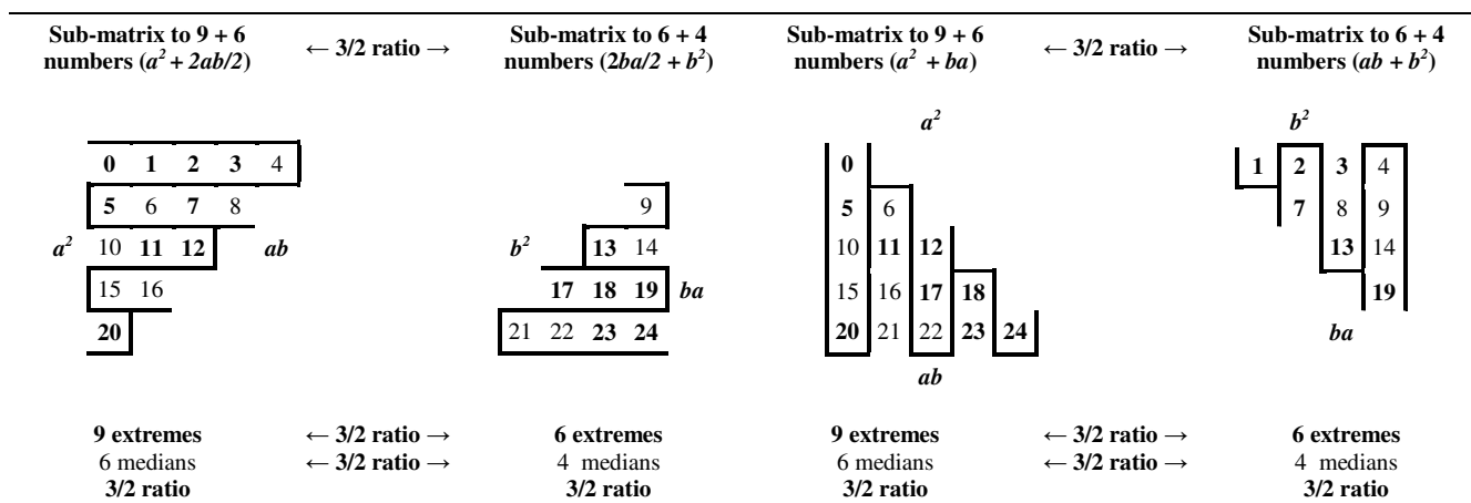
Fig. 57 Distribution of the numbers to extreme and median classes in two double sub-matrices of the first 25 numbers. Configurations inferred from the identity (a + b) \dots . Distribution des nombres de classes extrêmes et médianes dans deux doubles sous matrices des 25 premiers nombres. Configurations déduites de l'identité (a + b) \dots .
