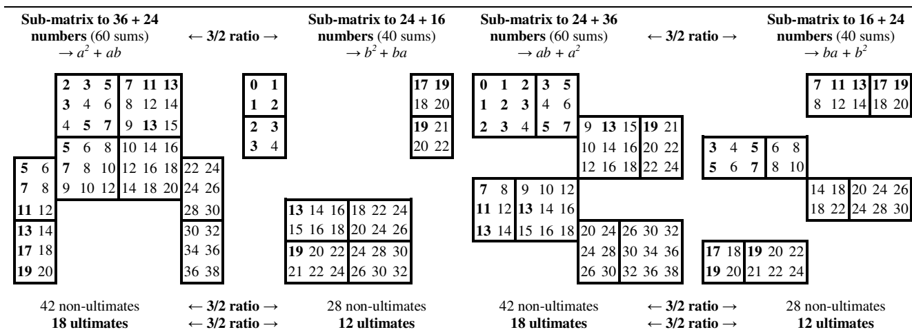
Fig.22 Addition sub-matrices of the ten primordial ultimates to 60 versus 40 numbers. Geometric variant of the remarkable identity (a + b)^2 = a^2 + 2ab + b^2 . Sous matrices d'addition des dix ultimes primordiaux de 60 contre 40 nombres. Variante géométrique de l'identité remarquable (a + b)^2 = a^2 + 2ab + b^2 .
