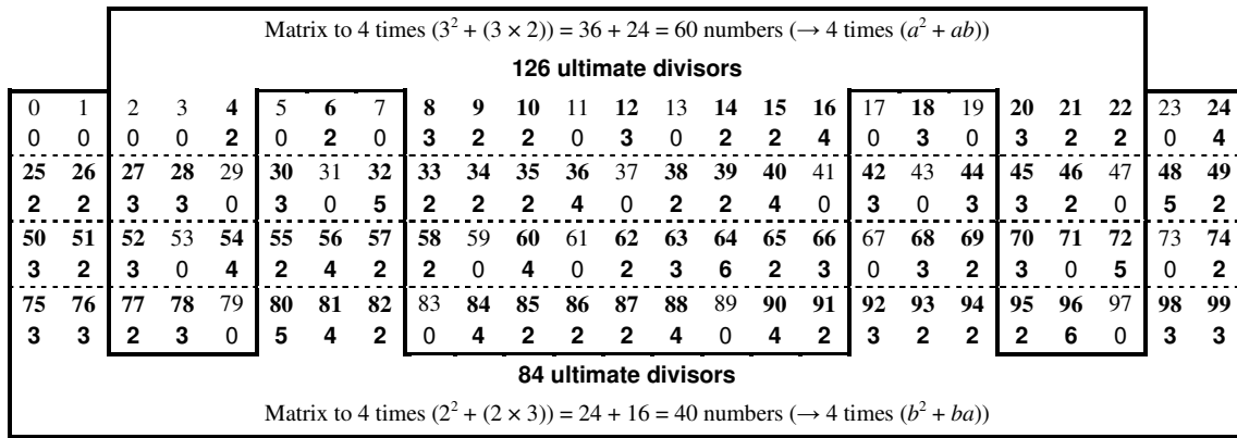
Fig. 49 Counting of the ultimate divisors in a redeployment of the matrix of the first 100 numbers registering in the remarkable identity (a + b)^2 = a^2 + 2ab + b^2 where a and b have as 3 and 2 to value. Distribution of the 210 divisors in 3/2 ratio in two entangled sub-matrices to 60 versus 40 entities. Décompte des diviseurs ultimes dans un redéploiement de la matrice des 100 premiers nombres s'inscrivant dans l'identité remarquable (a + b)^2 = a^2 + 2ab + b^2 où a et b ont les valeurs 3 et 2. Distribution des 210 diviseurs en ratio 3/2 dans deux sous matrices intriquées de 60 contre 40 entités.
