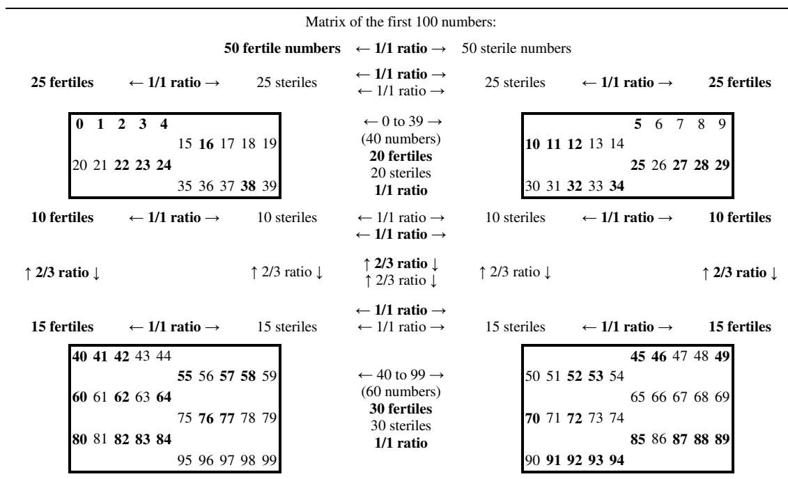
Fig. 73 Distribution of the 50 fertile numbers and the 50 sterile numbers in sub-matrices from the matrix of the first 100 numbers. Distribution des 50 nombres fertiles et des 50 nombres stériles dans des sous matrices issues de la matrice des 100 premiers nombres.
