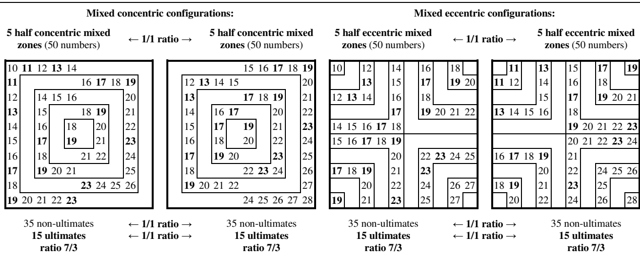
Fig. 14 From the addition matrix of the twenty fundamental numbers, concentric and eccentric configurations of sub-matrices to 50 entities each opposing their non-ultimates and their ultimates in 1/1 ratios. Depuis la matrice d'additions des vingt nombres fondamentaux, configurations concentriques et excentriques mixtes de sous matrices de chacune 50 entités opposant leurs non ultimes et leurs ultimes en ratios 1/1.
