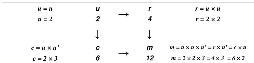
Fig. 39 Illustration of the concepts of ultimate numbers, ultimate divisors and ultimate algebra. Illustration des concepts de nombres ultimes, de diviseurs ultimes et d'algèbre ultime.
