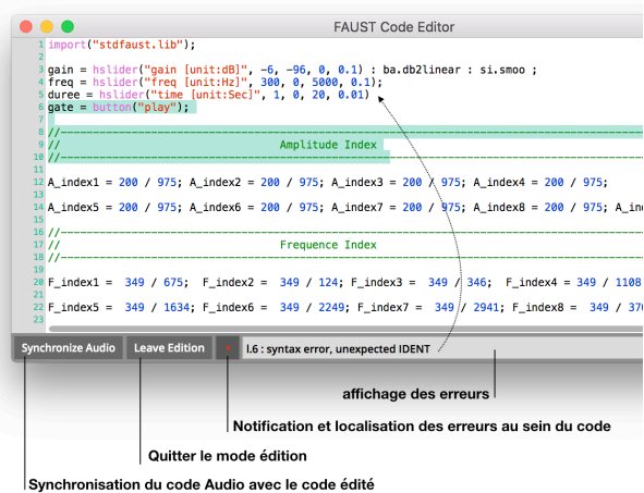
Figure 5. Interface graphique de l'éditeur de code Faust embarquée au sein de l'objet faust~ de Kiwi. La partie de code exposée dans cette capture provient d'une mise en œuvre en langage Faust du modèle de cloches de Risset, réalisée par le compositeur João Svidzinski.
