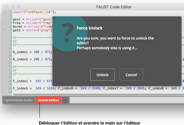
Figure 6. Interface graphique de l'éditeur de code de l'objet faust~ , tel qu'il apparaît à un utilisateur lorsque quelqu'un d'autre est en train d'éditer le texte. Le bouton « Unlock Edition » permet de prendre la main sur l'éditeur.
