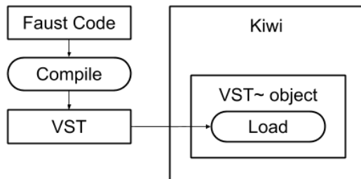
Figure 2. Schéma représentant la deuxième approche envisagée pour utiliser du code Faust au sein de l'application Kiwi. Le code Faust est compilé en un plugin VST qui est chargé dynamiquement dans Kiwi par un objet natif VST~ .
