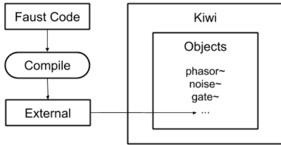
Figure 1. Schéma représentant la première approche envisagée pour utiliser du code Faust au sein de l'application Kiwi. Le code Faust est compilé en un objet externe Kiwi qui est intégré aux objets natifs de l'application.
