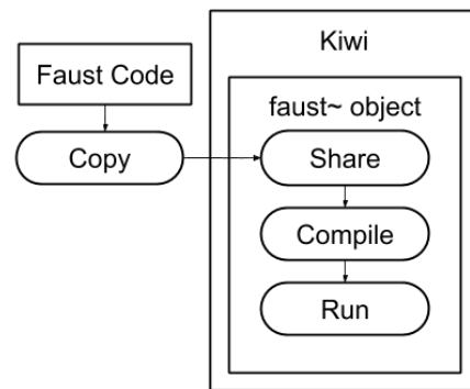
Figure 3. Schéma représentant l'approche finale pour utiliser du code Faust au sein de l'application Kiwi. Le code Faust est chargé et compilé dynamiquement dans Kiwi par un objet natif faust~ .
