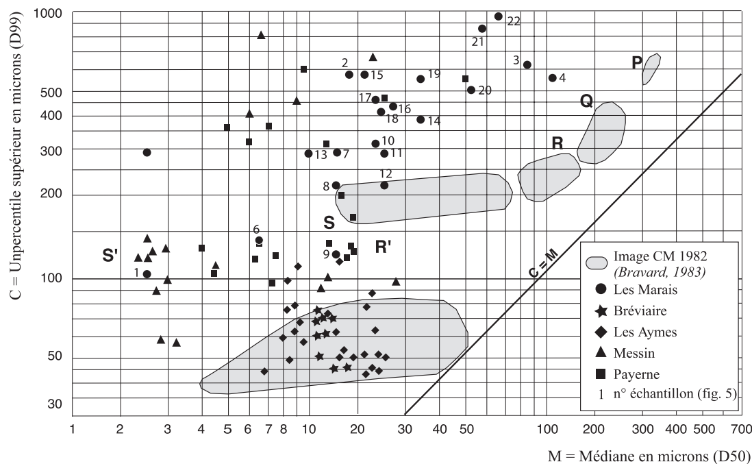
Fig. 3 : Les processus d'alluvionnement dans les paléochenaux, selon l'image CM. PQ : suspension graduée avec quelques grains roulés ; QR : suspension graduée ; RS : suspension uniforme en mode énergétique ; R'S' : suspension uniforme en mode calme.
