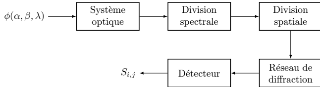
FIGURE 1 – Diagramme du modèle instrument
