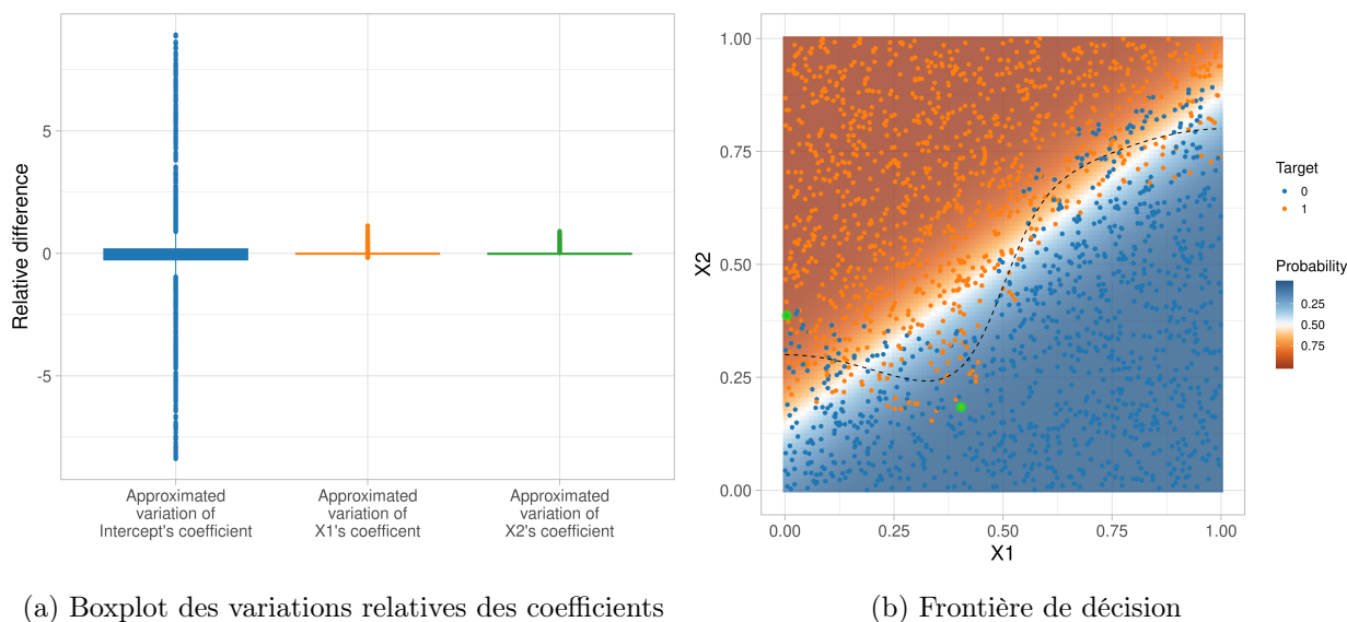
Figure 5 – Variation des coefficients d’une régression logistique consécutive au retrait d’un point de D_{train}
