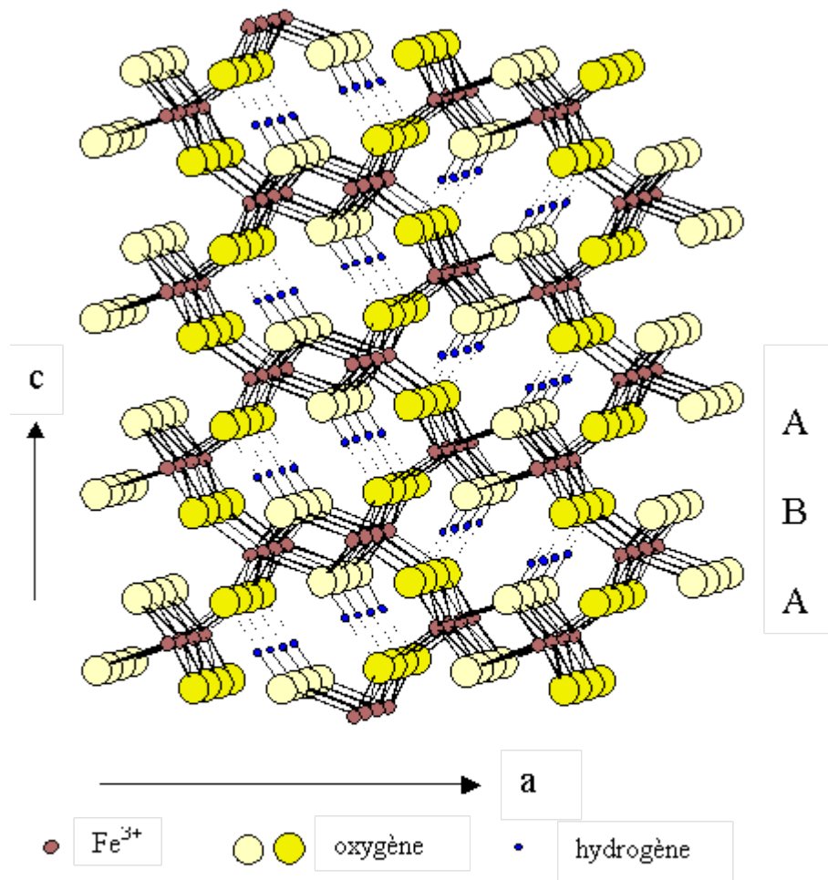
Figure 10 : Structure de la goethite \alpha -FeO(OH)
