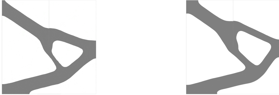
Figure 3: Forme optimisée avec l'approche "Ersatz" (gauche) et remaillage conforme (droite)
