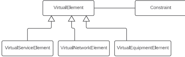
Fig. 1. VirtualElement Model
