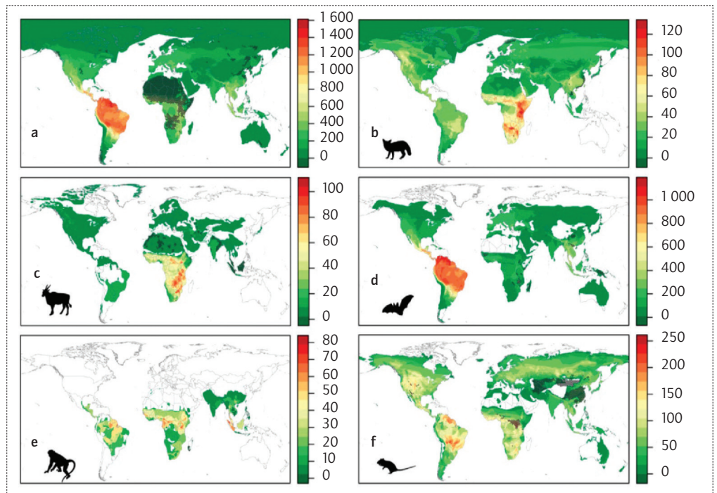
Figure 2 : Distribution attendue de nouvelles espèces de virus d'origine animale qu'il reste à découvrir par grands groupes taxonomiques animaux. a) Tous mammifères confondus ; b) Carnivores ; c) Cetartiodactyles ; d) Chiroptères, ou chauves-souris ; e) Primates ; et f) Rodentia, ou rongeurs. Les aires qui apparaissent en gris sont des zones pour lesquelles les modèles statistiques développés dans l'étude conduisent à des résultats biaisés. D'après Olival et al. (2017). © Nature. doi: 10.1038/nature22975
