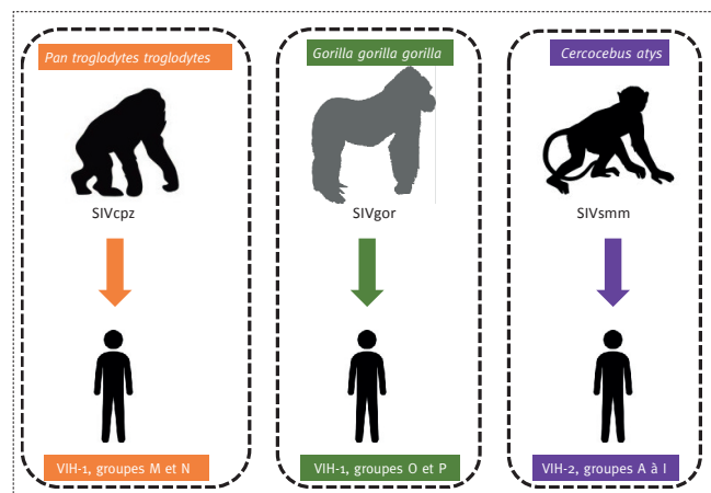
Figure 4 : Illustration des passages des virus d'immuno-déficience simiens (VIS, ou SIV en anglais) du chimpanzé, du gorille des plaines et du mangabé enfumé vers l'humain, donnant naissance aux différents groupes de virus d'immuno-déficience humains actuels.
