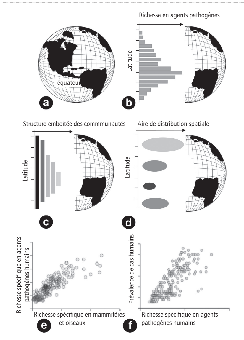
Figure 3 : Quelques patrons macro-épidémiologiques des agents microbiens et parasitaires affectant les populations humaines. Modifié d'après Murray et al. (2018).
