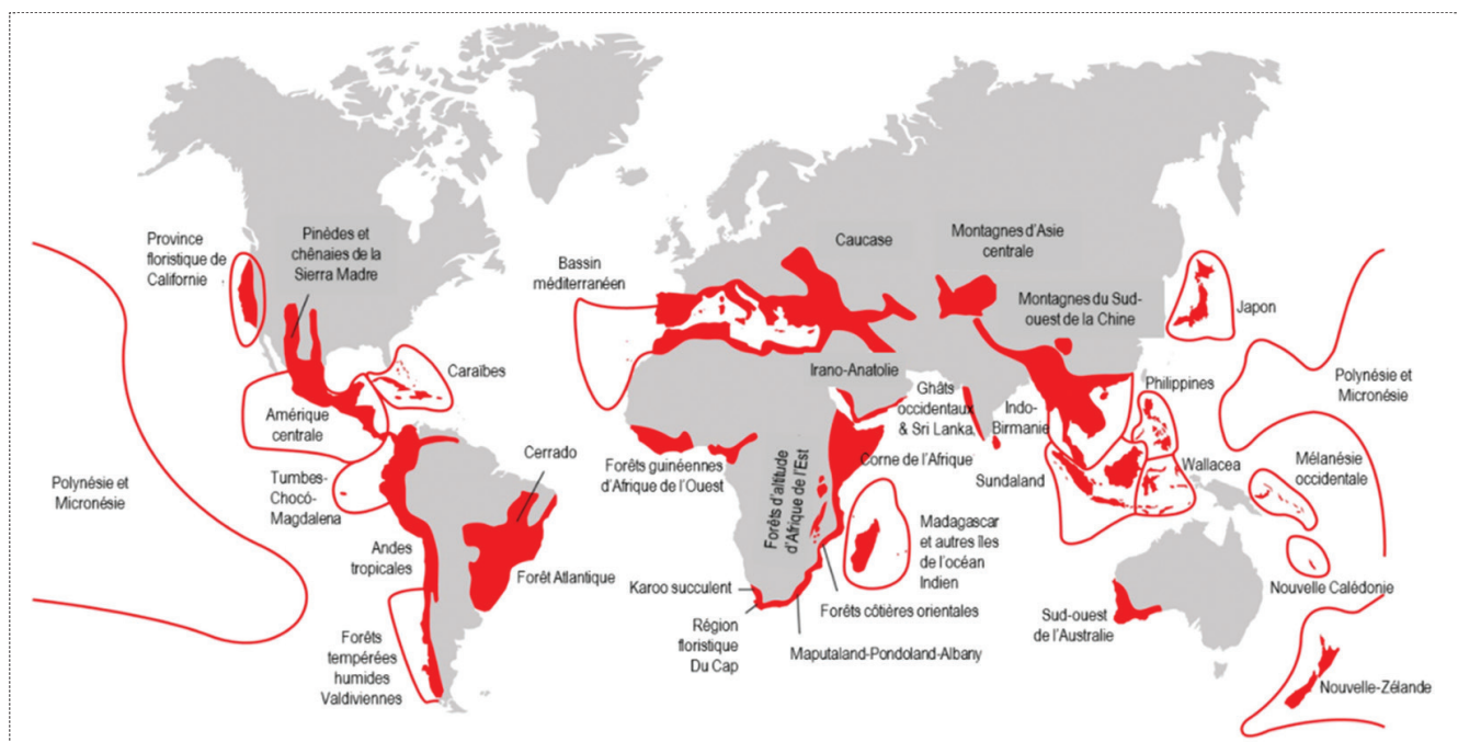
Figure 1 : Les « points chauds » de la biodiversité hébergent 70 % de toutes les espèces de plantes vasculaires connues, 35 % des vertébrés terrestres connus et 75 % de toutes les espèces considérées comme menacées. D'après Joyard (2017) [7], modifié de Jenkins et al. (2013) [8]
