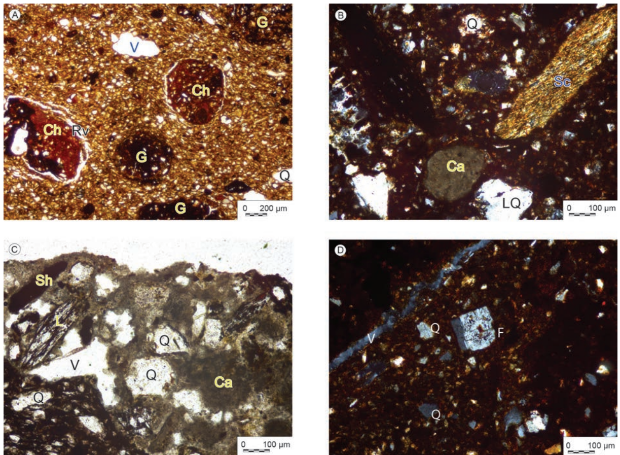
Fig. 34 – Lames minces en lumière naturelle ( A et C ) et en lumière polarisée ( B et D ). Ca , calcaire ; Ch , chamotte ; F , feldspath ; G , argile ferrique ; L , schiste micacé ; LQ , quartzite ; Q , quartz détritique ; RC , ringvoids ; Sc , schiste ; Sh , shale ; V , vide. A et B , brique de FAL (n° analyse BAV-23) ; C et D , briques d'ATIL (n°s analyse BAV-27 et 28) (clichés : É. Goemaere, Service géologique de Belgique).
