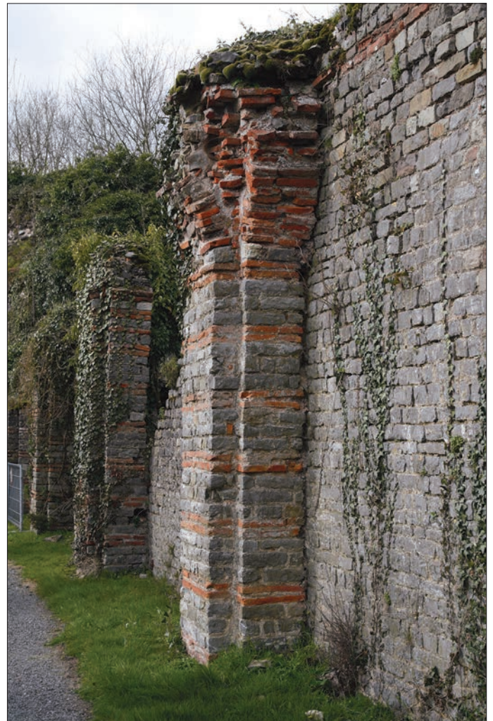
Fig. 8 – Le mur externe MCE32 conservé du premier forum, les demi-piliers PSE31-32 (fait architectural 20 ; technique A) surmontés de leur tas de charge (fait architectural 23 ; technique T) dans la branche septentrionale du cryptoportique (cliché : C. Louvion).
