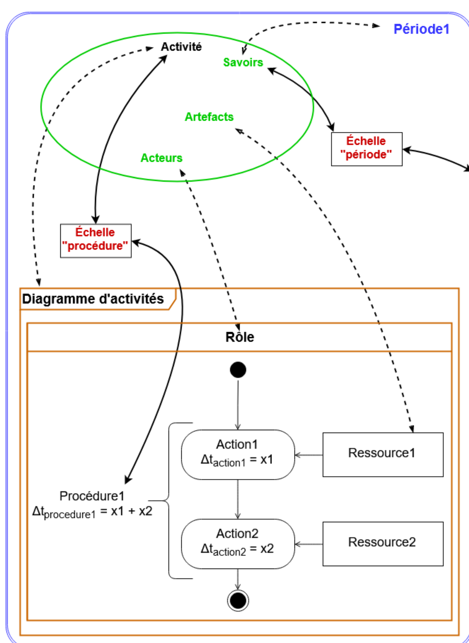
Modélisation de la représentation du temps (notions de Période , Procédure et Durée ) dans une activité par alignement entre ANY-Artefact [5] et MASCARET [1]
