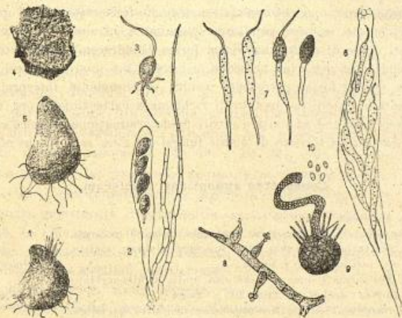
Fig. 87. 1-3. Podospora pasicea : 1 perithecium, 2 ascus, 3 sporidium. 4-10. Pod. coprophila : 4 habitus fungi, 5 perithecium, 6 ascus immaturus, 7 sporidia varie evoluta, 8 status conidicus, 9 status pycnidicus: pycnidium, 10 sporulae.
