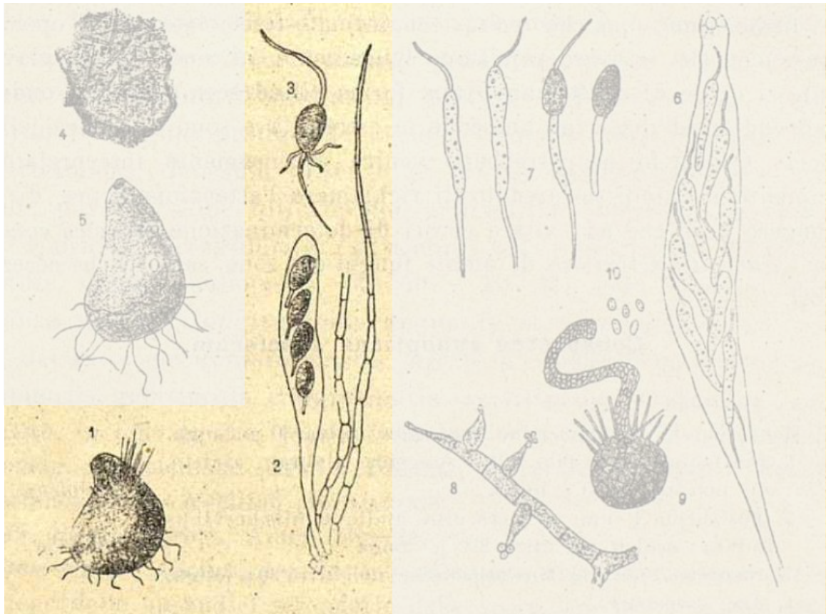
Fig. 87. 1-3. Podospora pauciseta : 1 perithecium, 2 ascus, 3 sporidium. 4-10. Pod. coprophila : 4 habitus fungi, 5 perithecium, 6 ascus immaturus, 7 spori- dia varie evoluta, 8 status conidicus, 9 status pycnidicus : pycnidium, 10 sporulae.
