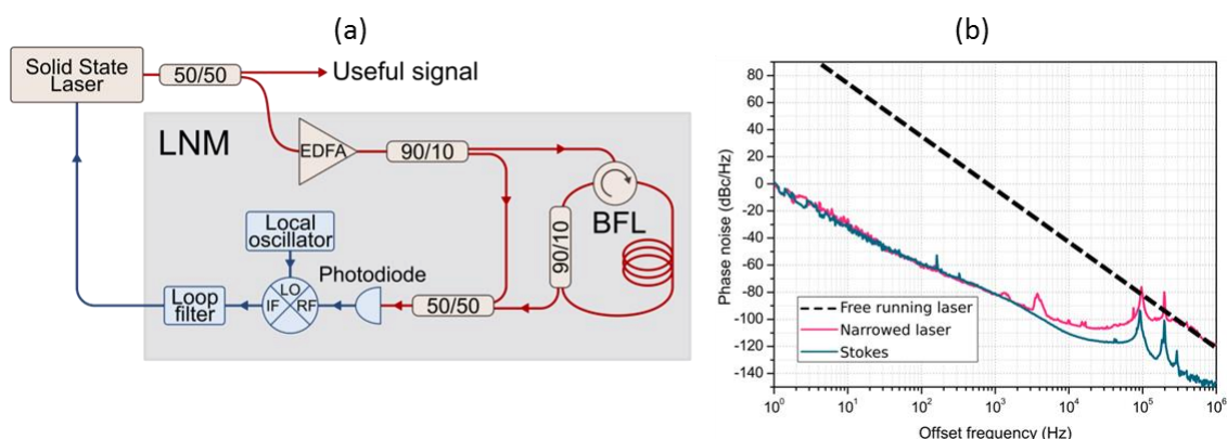
Figure 1. (a) Schéma du module de réduction de largeur de raie (LNM). OL : oscillateur local, RF : signal de battement, IF : fréquence intermédiaire. (b) Bruit de phase du battement entre deux lasers Er:Yb :verre stabilisés (courbe rose) et entre les ondes Stokes associées (courbe bleue). Ligne pointillée : bruit de phase optique typique de nos lasers Er:Yb : verre en régime non asservi.
