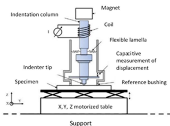
Figure 3 : Schéma de principe d'un nanoindenteur
