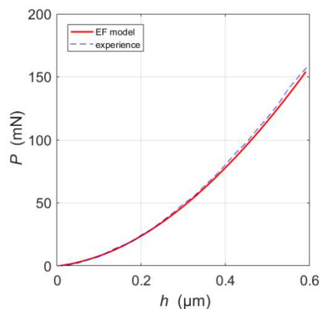
Figure 8 : Comparaison modèle-experience lors de l'enfoncement de la pointe c) Revêtement TiAl et d) Revêtement TiAlN
