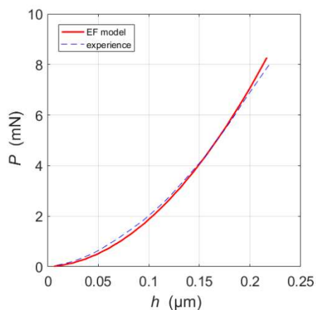
Figure 8 : Comparaison modèle-experience lors de l'enfoncement de la pointe c) Revêtement TiAl et d) Revêtement TiAlN
