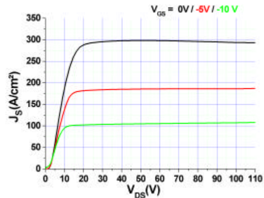
Fig. 7 I DS (V DS ) versus gate to source applied voltage.
