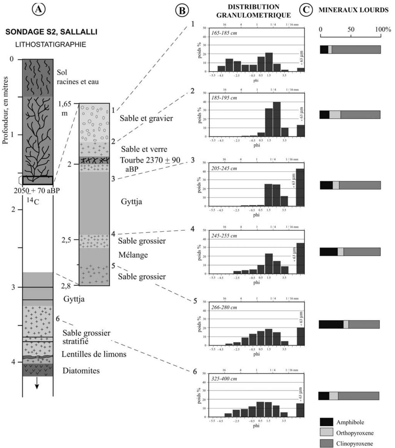
Fig. 5 : A. Lithostratigraphie de la carotte du sondage S2 ; B. Distribution granulométrique des couches minérales ; C. Minéraux denses de plus de plus de 105 \mu\text{m} des mêmes couches.
