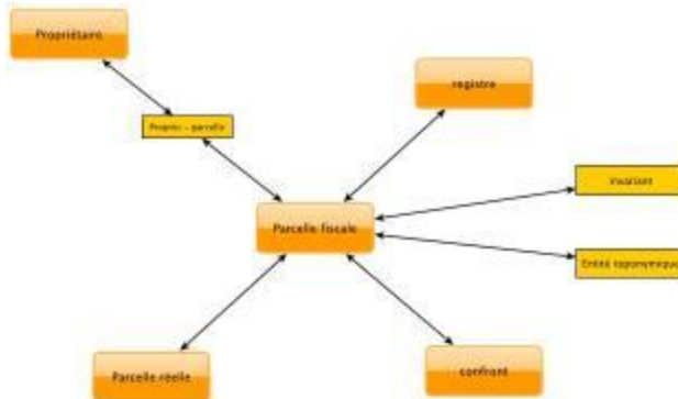
FIG. 4 - Schéma relationnel simplifié de la base de données TERCOMP.
