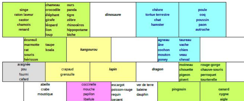
FIG. 1 – Clustering des animaux : carte auto-organisatrice de Kohonen (maillage hexagonal, dimensions : 5×4).
