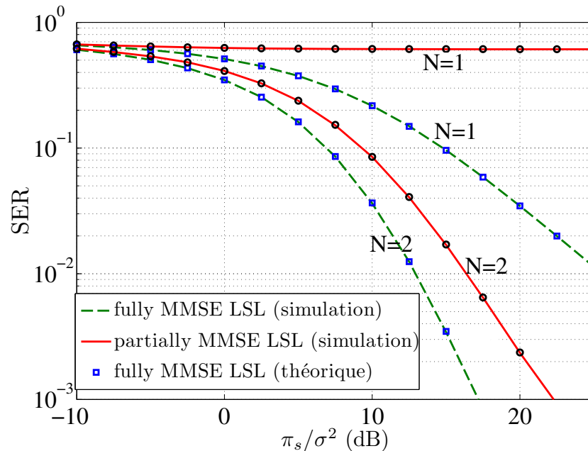
Figure 6. Comparaison des SER pour N = 1 et N = 2
