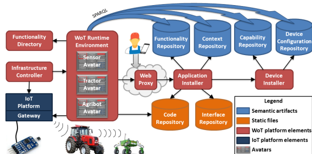
FIGURE 3 – Architecture d'une plateforme orientée-avatar pour le WoT.
