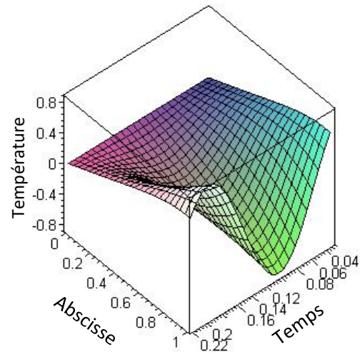
Figure 6. Pastille avec alimentation adiabatique ( h=0 )
