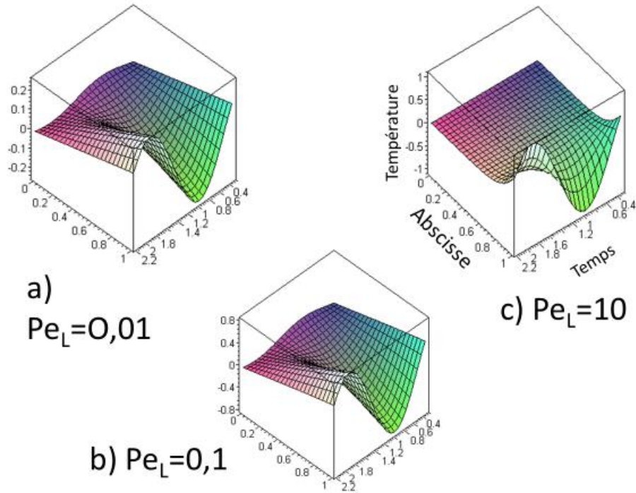
Figure 5. Influence du nombre de Péclet Pe_L (inverse de \theta ) pour des valeurs identiques des autres paramètres \varepsilon=1 , h=10 , u=10 , A=10 , B=100 Les axes correspondent à des coordonnées réduites : température X=T'_{l\text{réd}} , abscisse \xi = x/x_s , temps \tau = t/\bar{\tau}_v .
