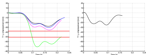
Figure 16. T1 y displacement NBDL (L), P&C.
