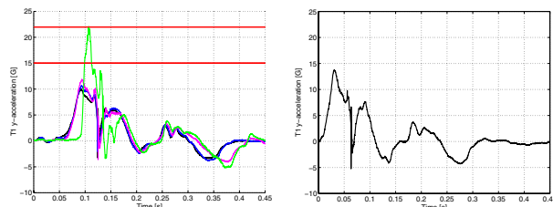
Figure 15. T1 y-acceleration NBDL (L), P&C.
