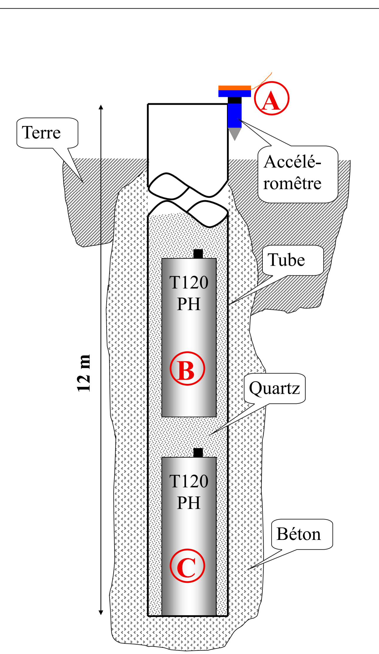
Schéma d'installation des différents capteurs pour les analyses.
